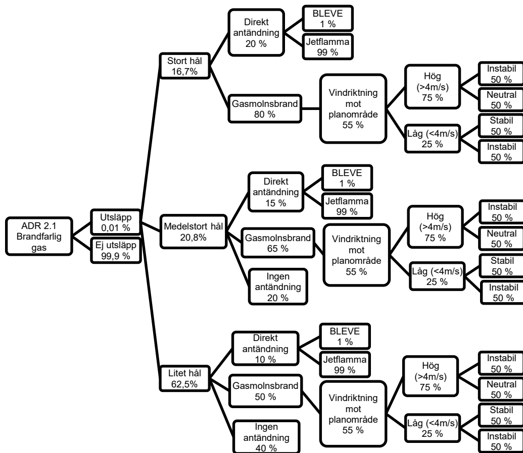
Figur 16. Händelsesträd för ADR-klass 2.1 – Brandfarliga gaser.
