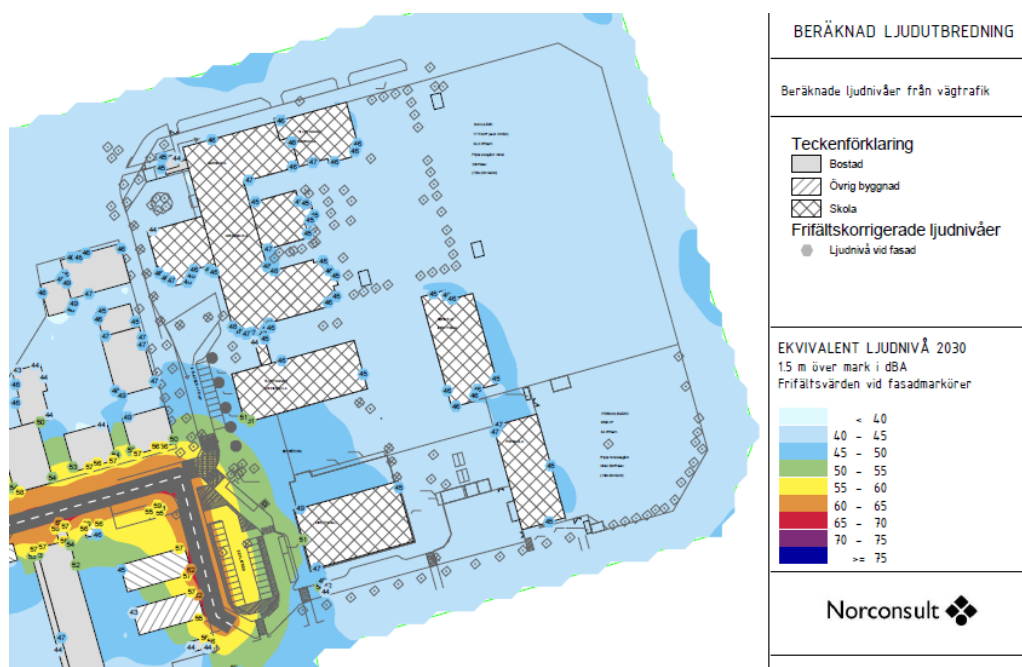
Figur 33 Ekvivalent ljudnivå 1,5 meter över mark, prognosår 2030.
