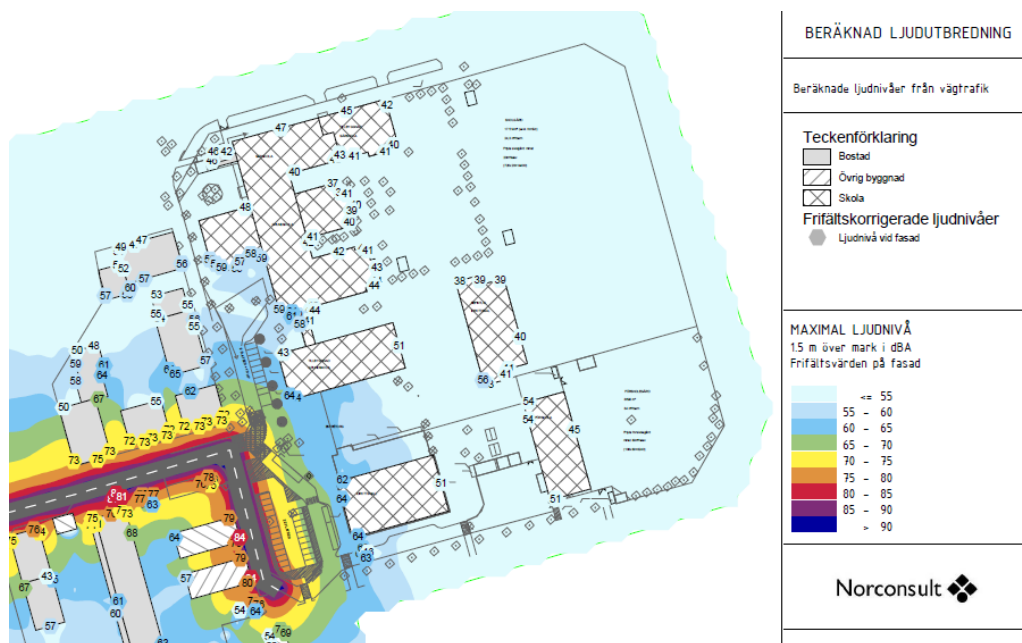
Figur 34 Maximal ljudnivå 1,5 meter över mark, prognosår 2030.
