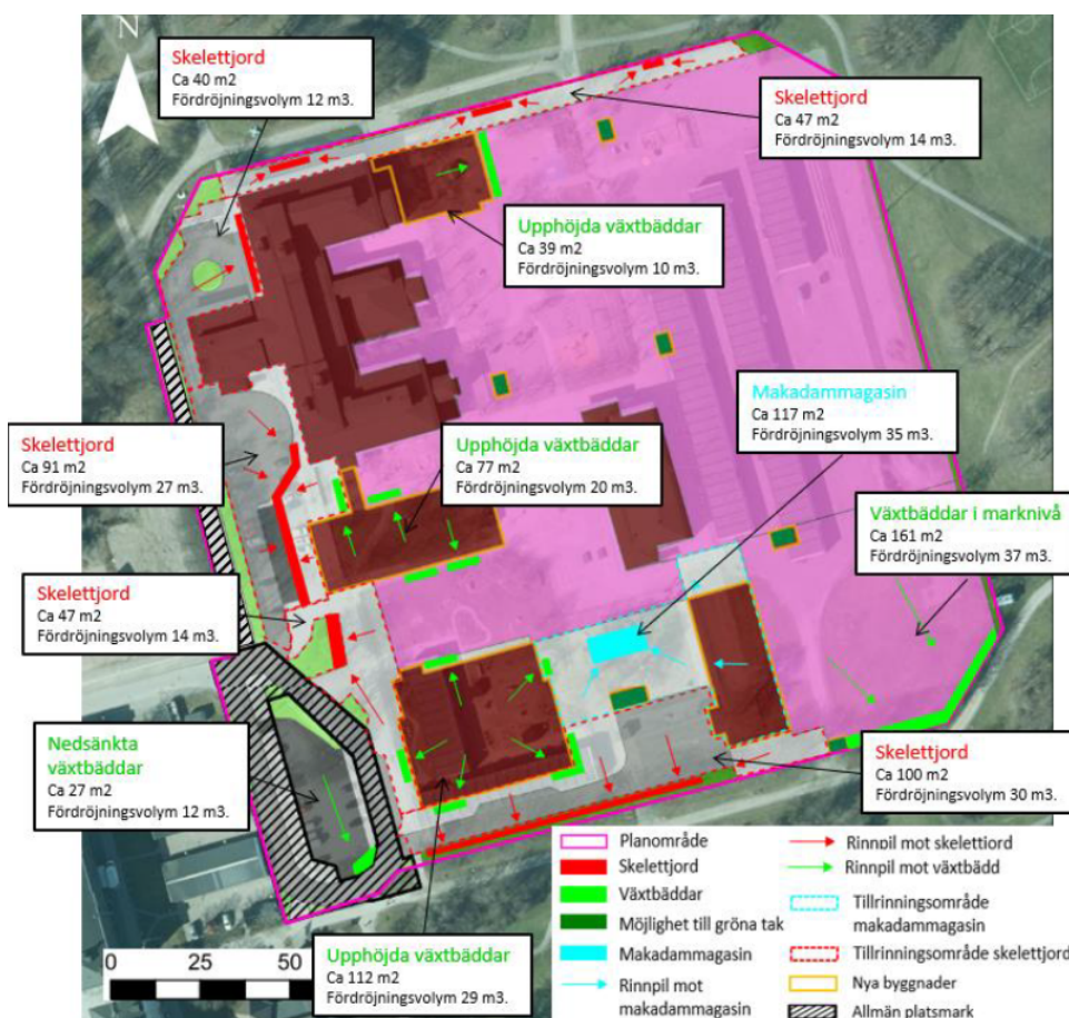
Figur 30 Föreslag på dagvattenhantering för kvartersmarken inom planområdet ur Bjerking's dagvattenutredning.
