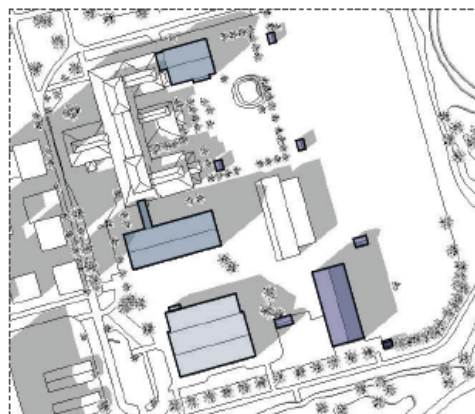
Vår/höstdagjämningen kl 15
