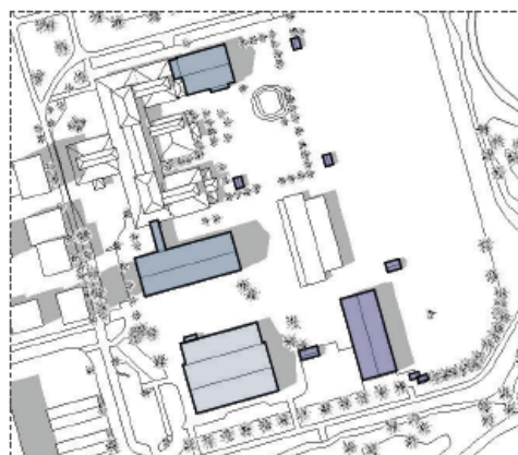
Sommarsolstånd kl 15
