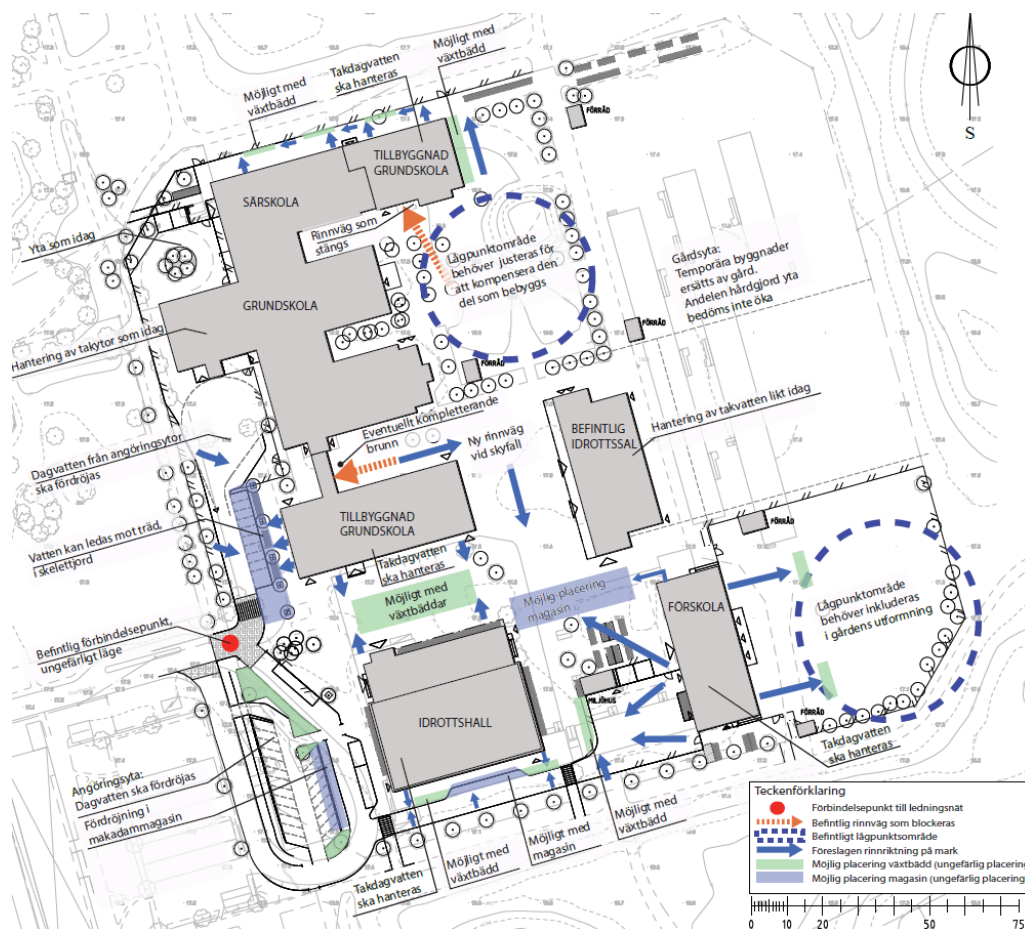
Figur 31 Föreslagen dagvattenprincip för kvartersmarken. Illustration av Ramboll.
