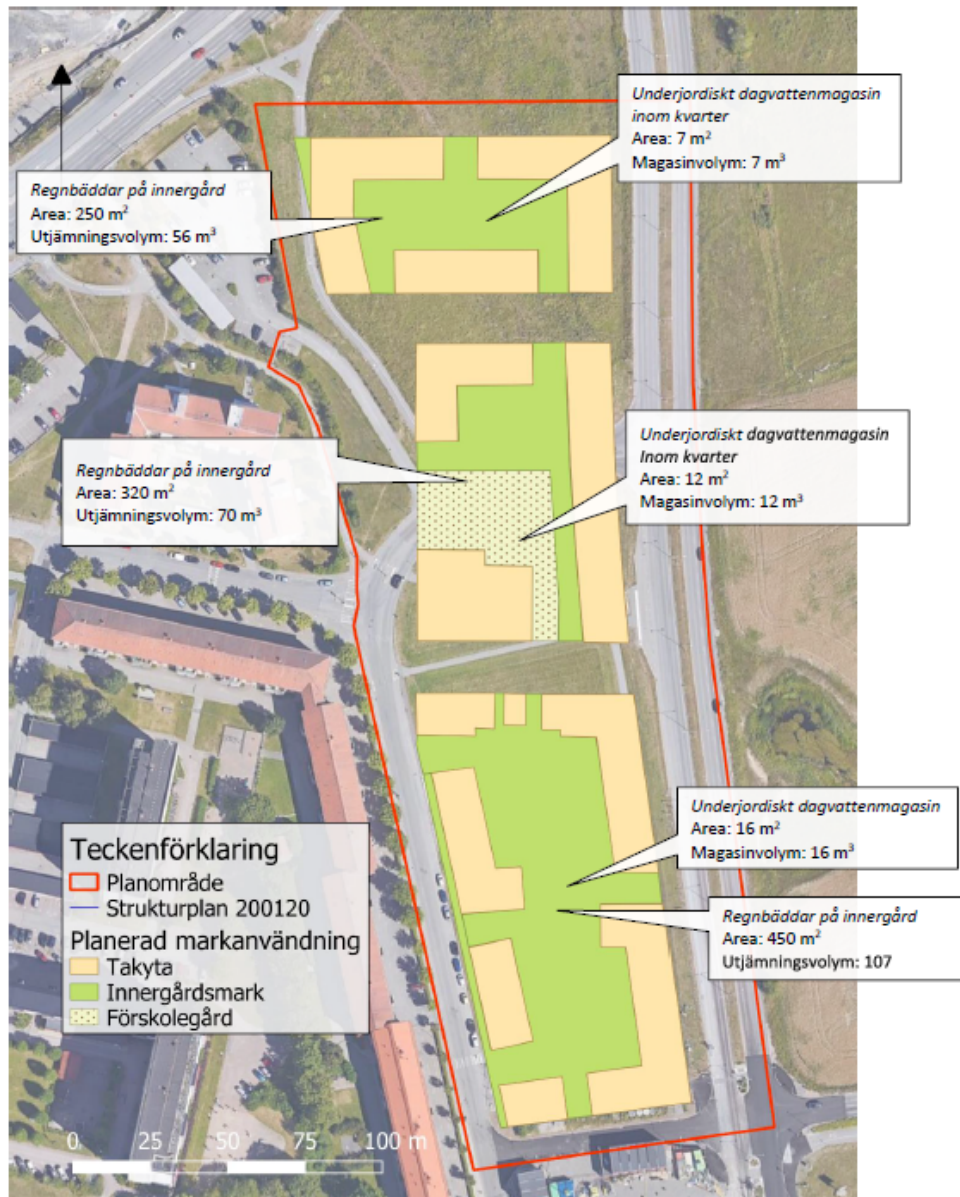
Lösningförslag för dagvattenhantering inom kvartersmarken i planområdet, Geosigma. Utöver dessa ytor kan dagvatten även hanteras inom förgårdsmarken längs lokalgatorna.
