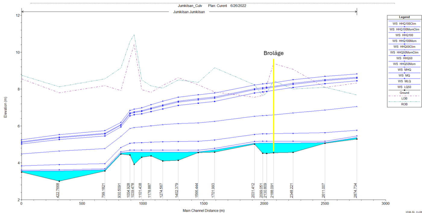
Figur 4: Beräknade vattennivåprofiler (blå linjer) för olika flöden (nedifrån räknat LLQ, MLQ, MQ, MHQ, HQ50 och HQ100) vid broläget. Svart linje visar bottennivåer i vattendraget och gul linje ungefärligt broläge.
