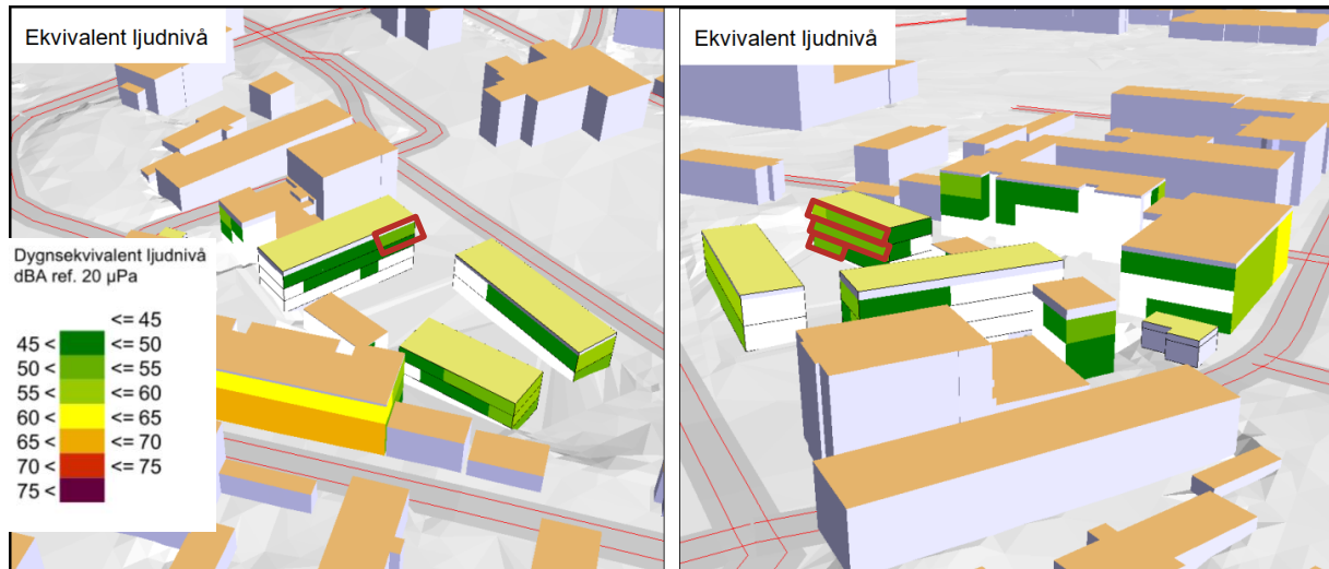
Figur 4. Här syns att de ekvivalenta ljudnivåerna överstiger 50 dBA ekvivalent ljudnivå på del av fasaden mot innergården på bostadsbyggnaderna.
