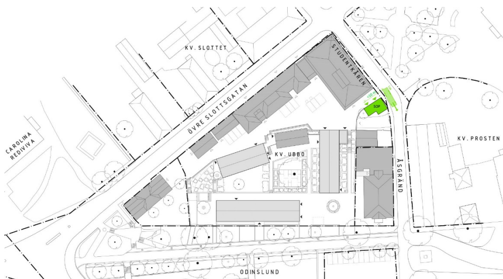
Figur 35. Illustration som visar placering av nytt sophus samt plats i gatan för hämtning av avfall. Bernow & Partner arkitekter.
