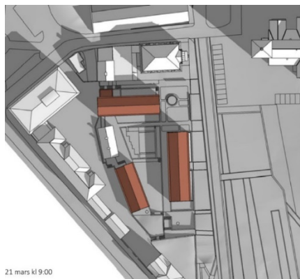
Figur 37. Sol och skuggstudie utan träd, 21 mars klockan 9 och 12, Bernow & Partners arkitekter
