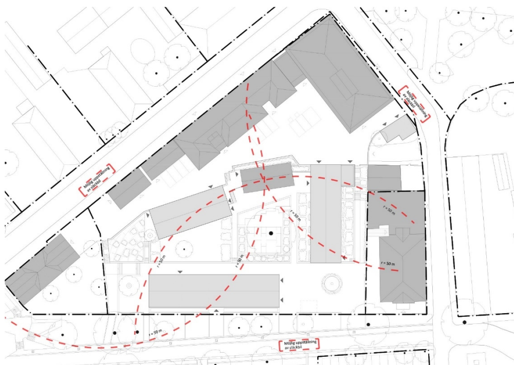
Figur 34. Illustration som visar uppställning av räddningsfordon och hur de kan nå byggnaderna på ett avstånd av högst 50 meter. Bernow & Partners arkitekter/Briab.
