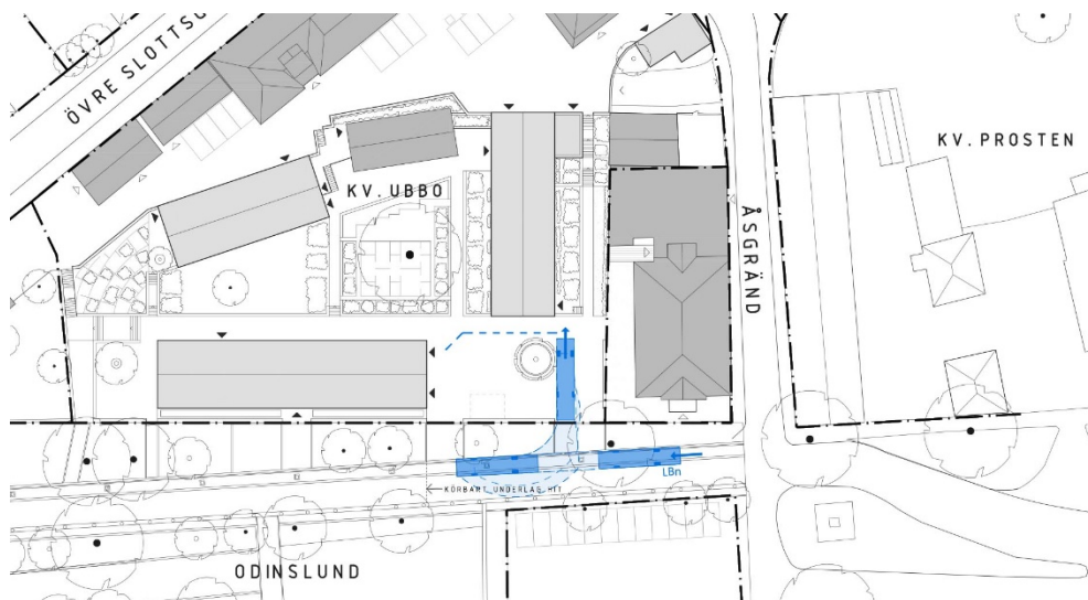
Figur 31. Illustration som visar hur varutransporter kan ske till hotellet Villa Anna. Bernow & Partners arkitekter.
