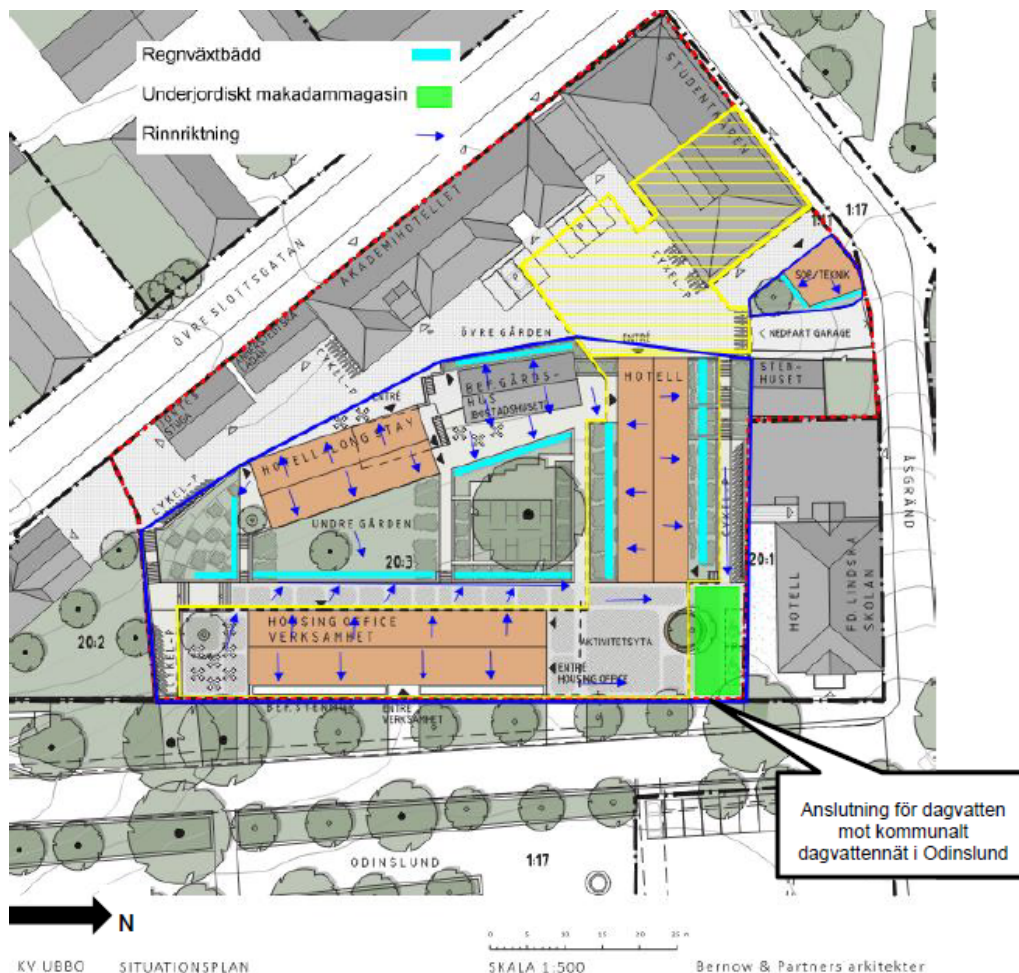
Figur 32. Illustration som visar hur dagvattnet rinner samt placering av regnväxtbäddar och underjordiskt magasin, Bjerking.
