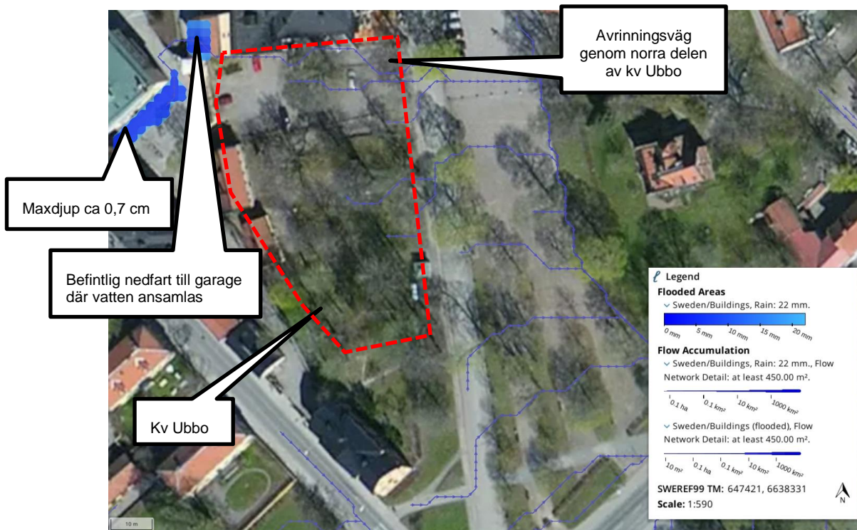
Figur 7. Ytliga avrinningsvägar vid 22 mm nederbörd inom och omkring utredningsområdet (rödsträckt område). Lågpunkten närmast utredningsområdet är i läget för en befintlig nedfart till ett underjordiskt garage. ©Lantmäteriet.
