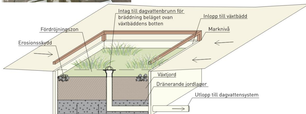
Figur 12. Exempel på upphöjd regnväxtbädd (överst) och nedsänkt regnväxtbädd med kupolbrunn och tät botten som medför att dagvatten kan stå ovan jordlagret och brädda mot ledningsnätet (nederst) (foto och illustration av Bjerking AB).
