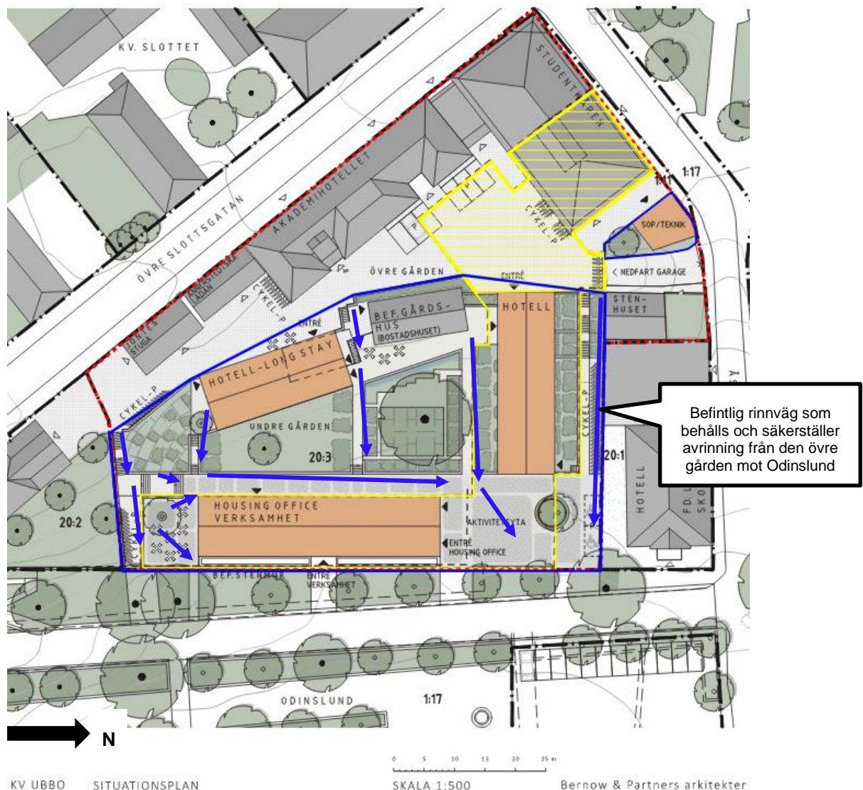
Figur 14. De sekundära avrinningsvägarna (blå pilar) inom kv Ubbo går mot Odinslund och vidare sydost, så som rinnvägarna går idag vid extrem nederbörd. Fastighetsgränsen visas med röd streckad linje, utredningsområdet med blå linje och underjordiskt garage/källare med gul linje.
