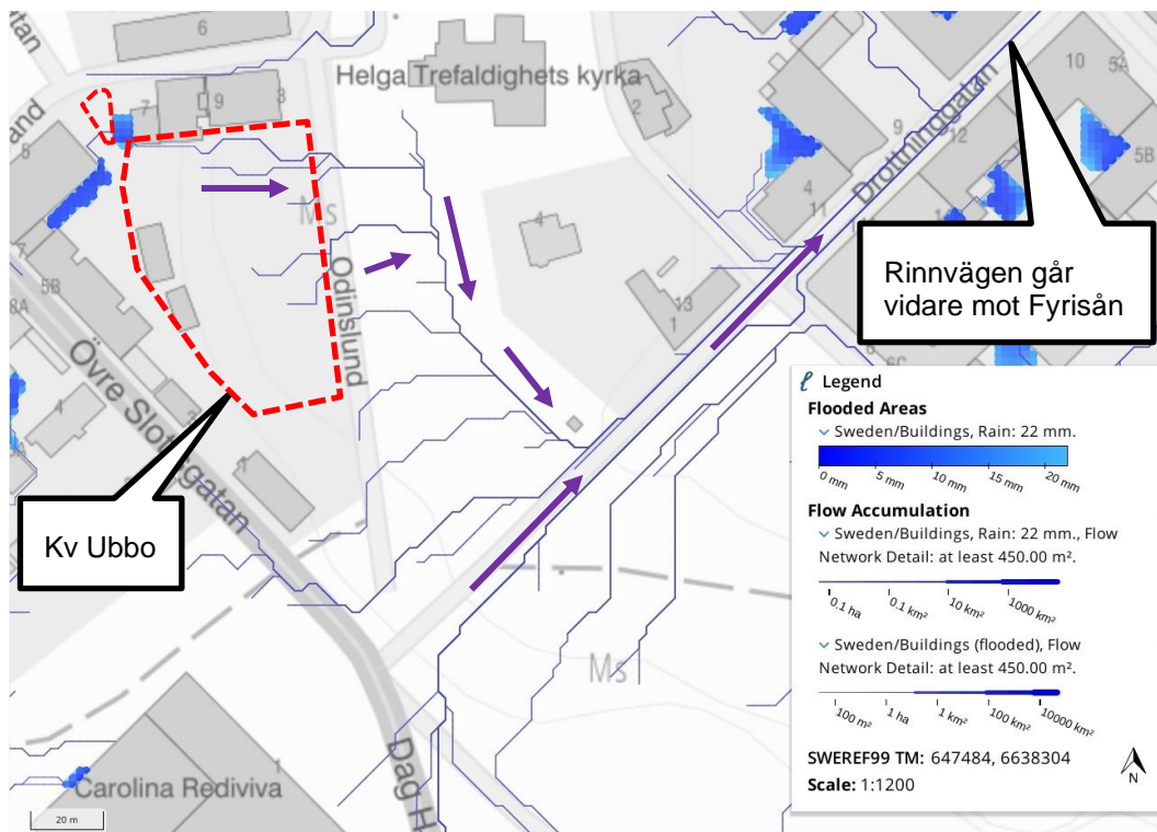
Figur 6. Ytliga avrinningsvägar (blå linjer) inom och omkring utredningsområdet (röd streckat område) för ett 20-årsregn under 10 minuter och klimatfaktor 1,25 (22 mm nederbörd). Blå områden visar områden där vatten ansamlas. Lila pilar påvisar avrinningsriktningen. ©Lantmäteriet.
