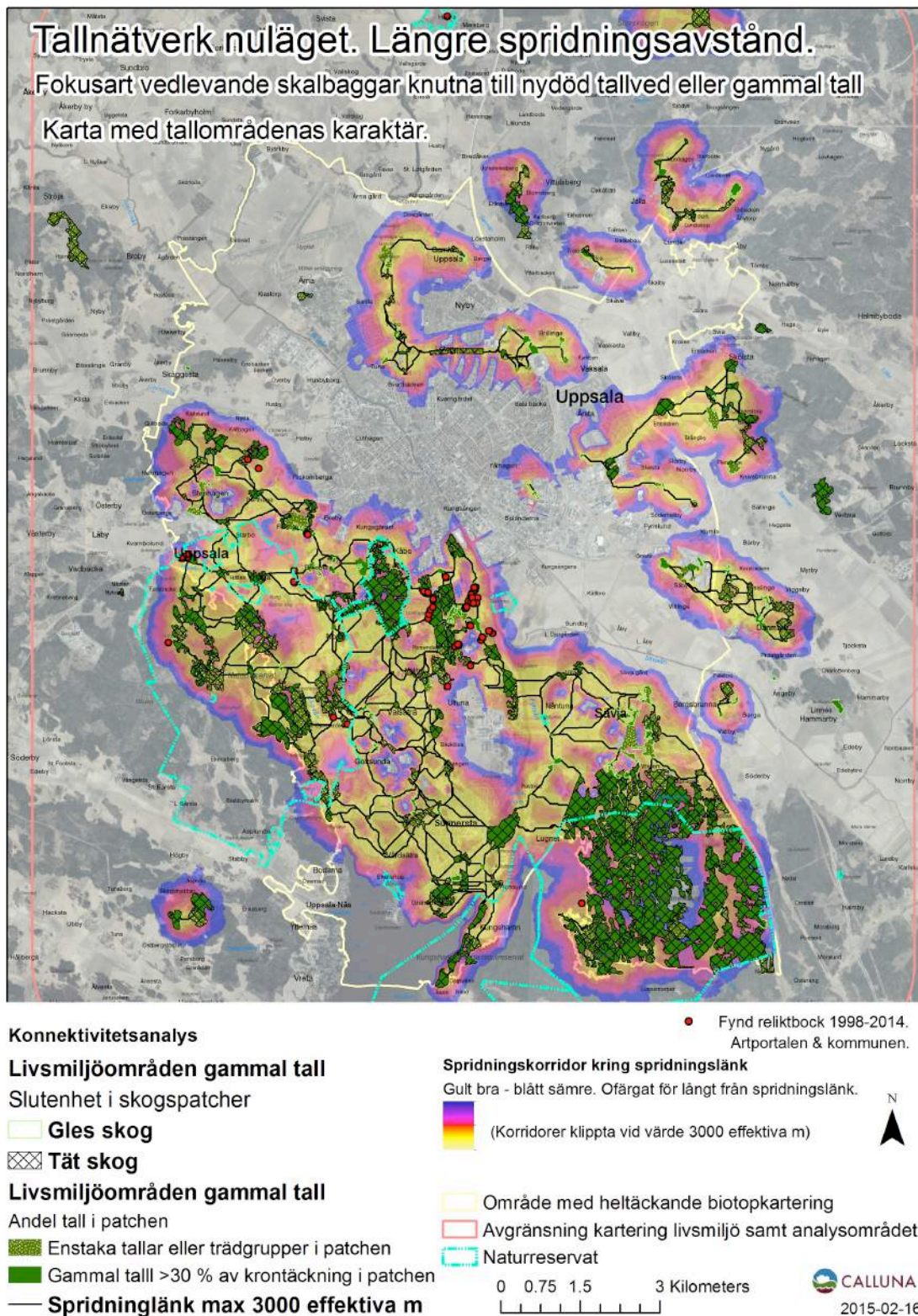
Figur 8. Tallnätverket gammal tall. Kartan är likadan som föregående karta, med skillnaden att här visas även karaktären på livsmiljöområdena. Klassningen gles eller tæt skog samt mängden gamla tallar, uppdelat i två klasser. (För bättre upplösning på kartan hänvisas till högupplösta kartor levererade till kommunen.)
