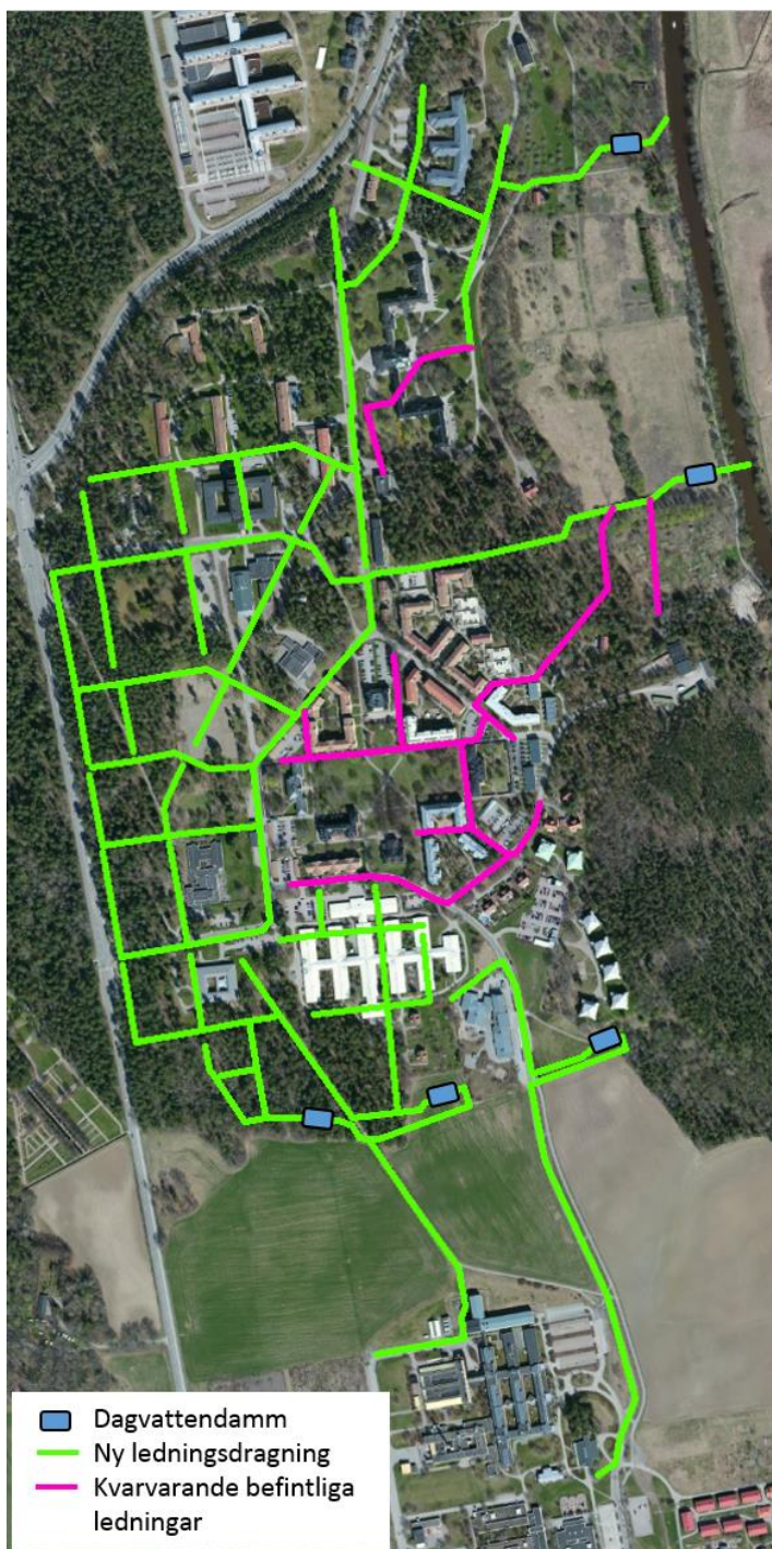
Figur 1: Befintligt och planerat ledningssystem för dagvatten samt placering av planerade dagvattendamm.
