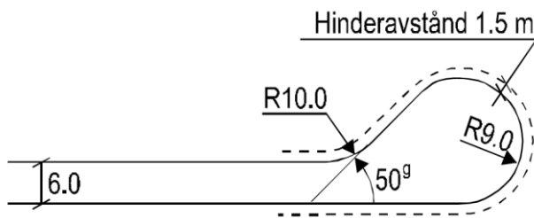
Figur 4.1-3. Minsta utrymme för vändmöjlighet (backvändning) typfordon LBn.
