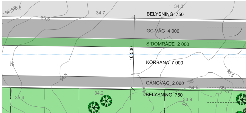
Figur 4.1-2. Gatusektion Siriusvägen.
