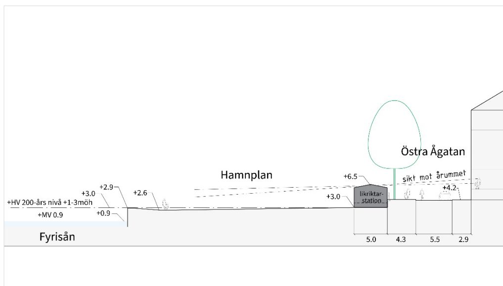
Bild 12. Sektion A-A (se bild 7) som visar likriktarstationens placering i förhållande till Fyrisån, Östra Ågatan och befintlig bebyggelse. Sektionen illustrerar också hur sikten från flerbostadshuset påverkas, vilket är ett motiv till att nockhöjden hålls nere så mycket som möjligt. Illustration: White arkitekter (bearbetad av stadsbyggnadsförvaltningen)
