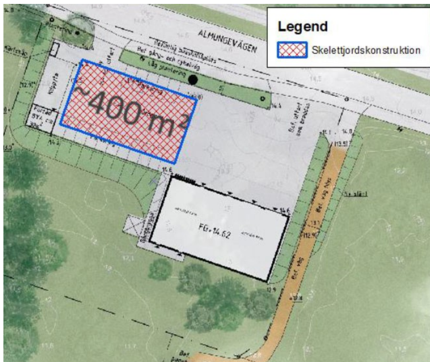
Utdrag ur dagvattenutredningen som visar ett möjligt läge för en skelettjordskonstruktion för omhändertagande av dagvatten, Sweco Architects AB.
