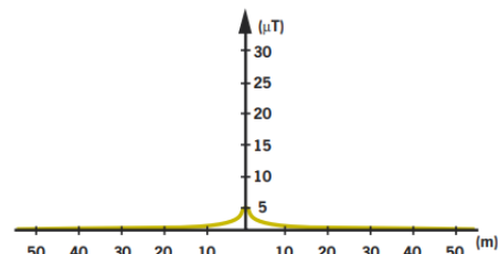
Magnetfältets styrka på olika avstånd från järnvägen när tåget är långt borta (mer än 2,5 kilometer bort). Strömstyrkan är 200 A och frekvensen 16,7 Hz.
