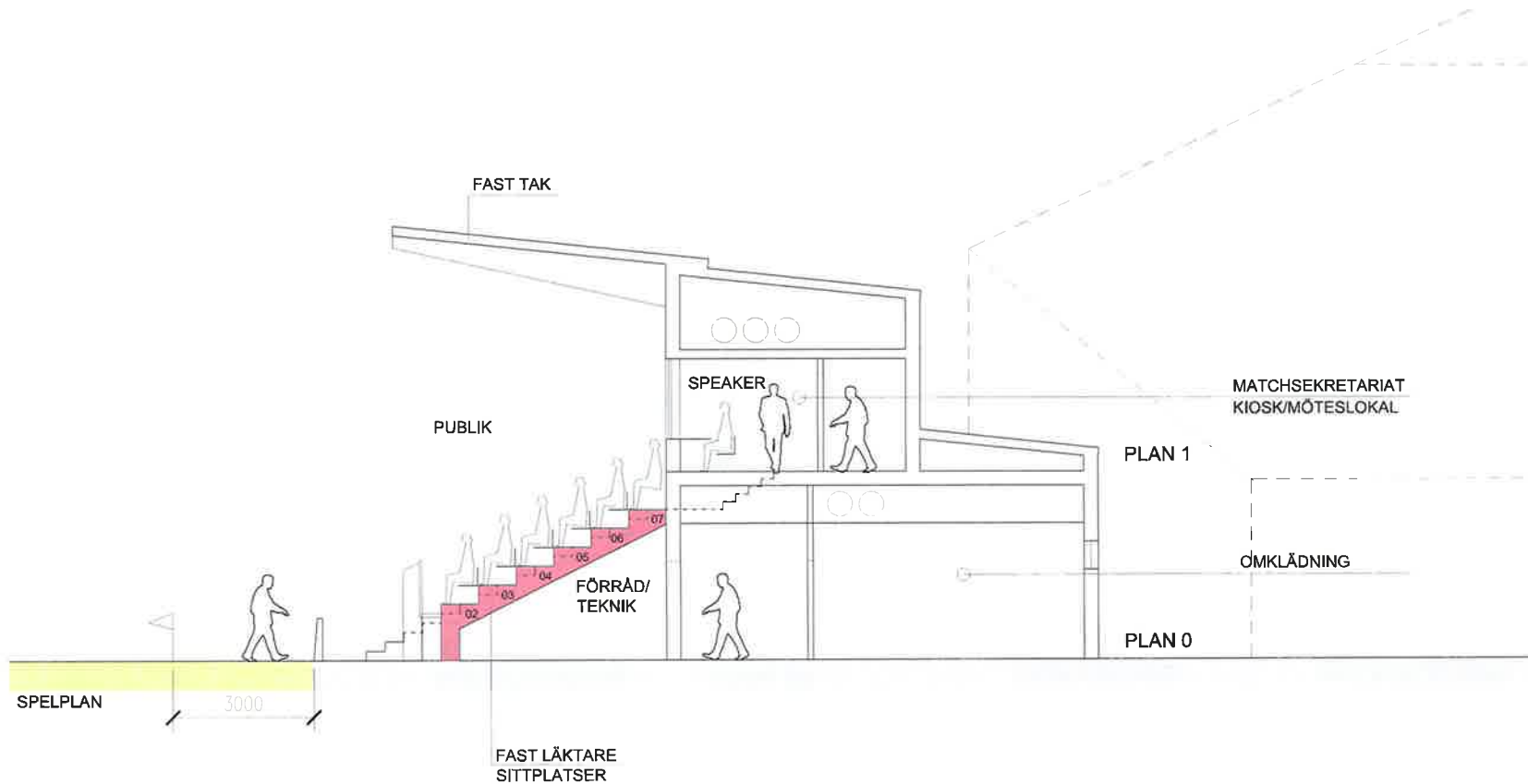
SEKTION A-A GENOM MITTSEKTION
