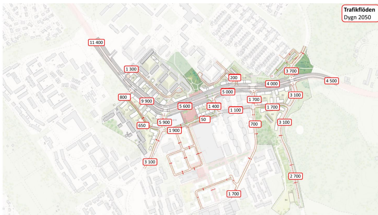
Figur 4 - Trafikflöden (ÅDVT), 2050
