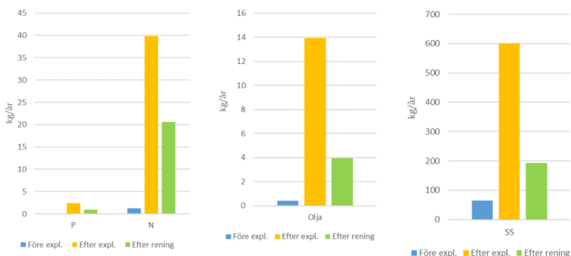
Figur 69. T.v. föroreningstransport (kg/år) av näringsämnena. Mitten: föroreningstransport av olja (kg/år). T.h. föroreningstransport (kg/år) av SS. Källa: (WSP, 2022b).
