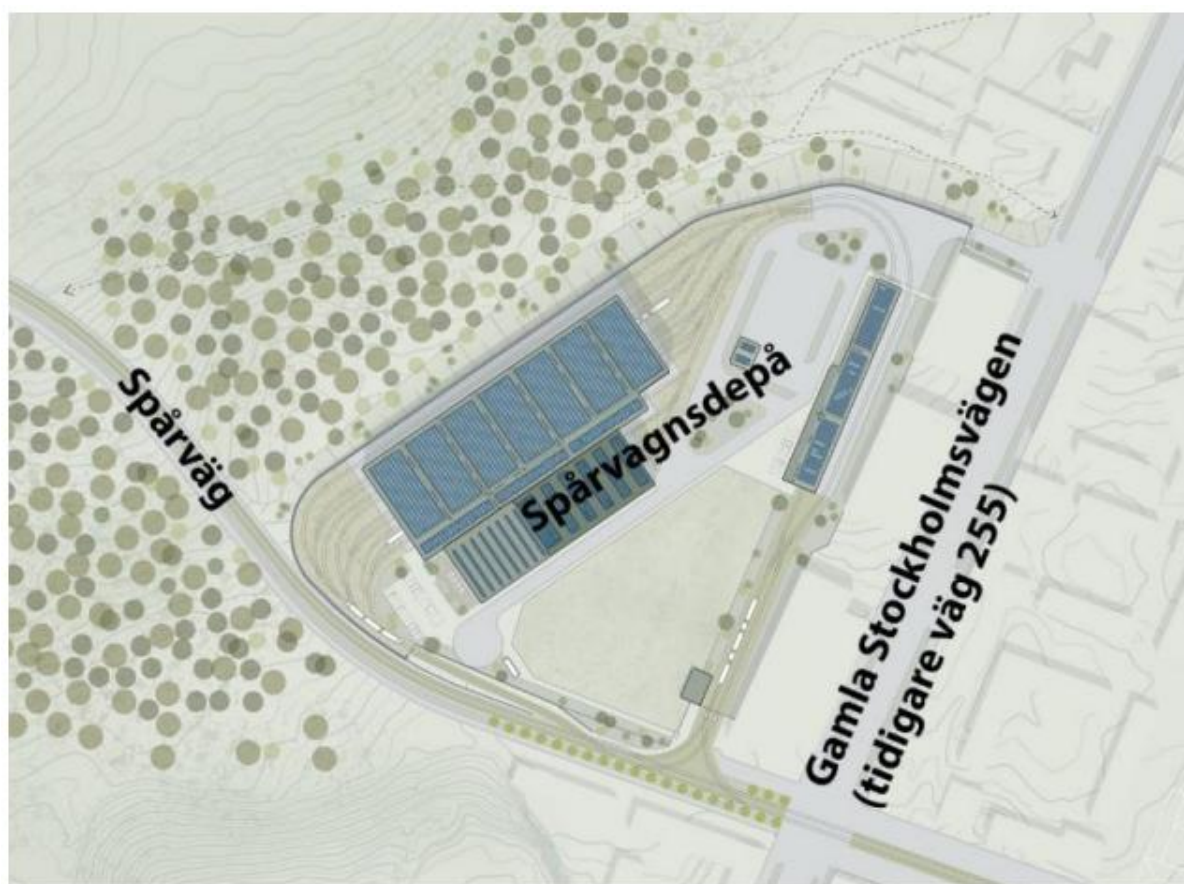
Figur 24. Situationsplan för spårvagnsdepå intill Gamla Stockholmsvägen (tidigare väg 255). Spårvägen passerar söder om depå. Bild: White arkitekter, redigerad av Uppsala kommun.
