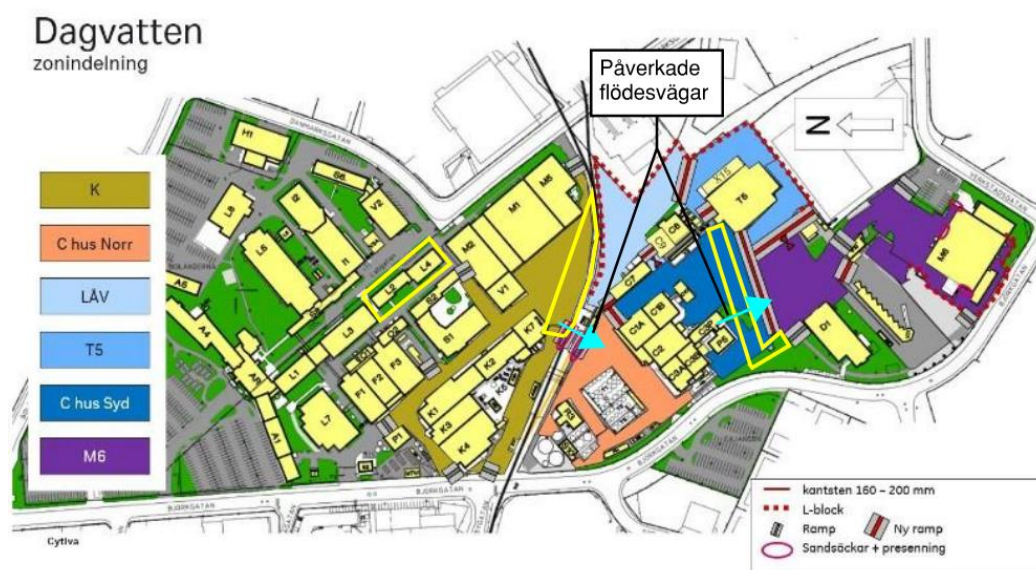
Figur 10. Påverkade rinnvägar för dagvatten (blåa pilar) i planområdet (gula linjer) bild från prøvotidsredovisningen. Cytiva 2021.
