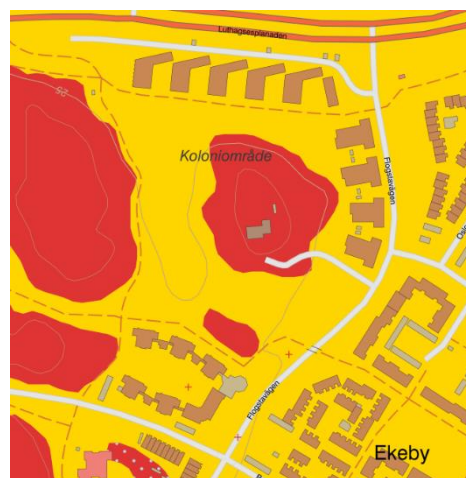
Figur 2. Jordartskarta. Gult färgat område visar glacial lera och rött färgat område berg i dagen.
