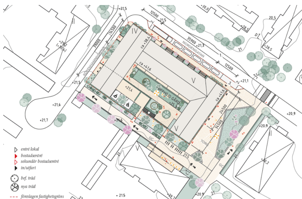
Bild 6 Situationsplan, DinellJohansson
