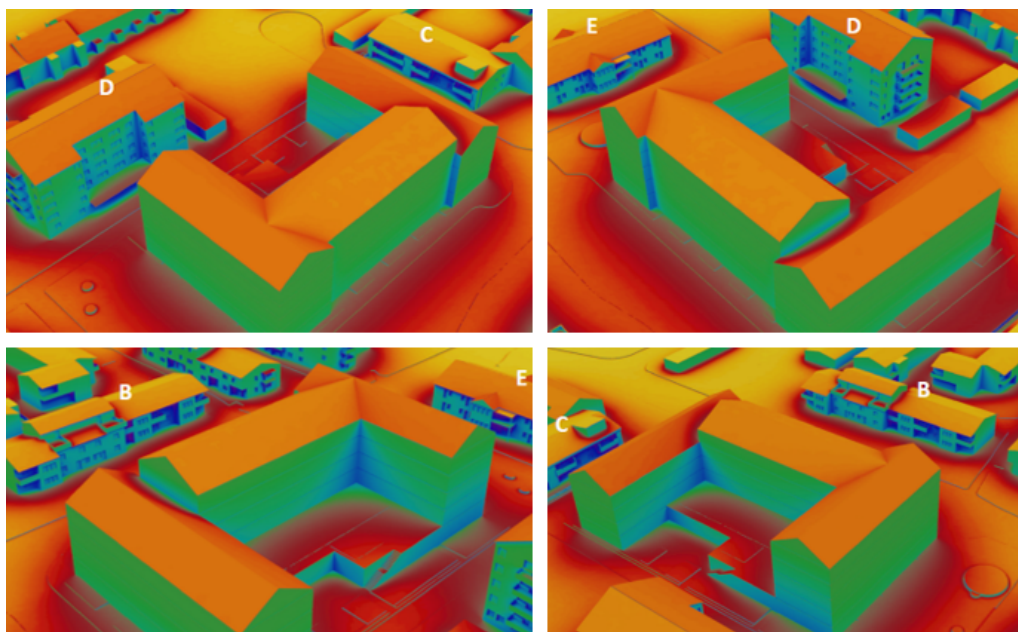
Bild 40 Tillgång till diffust dagsljus på fasad hos den föreslagna bebyggelsen. Mörkblå färg indikerar att särskilda anpassningar kan behöva göras fr att uppnå dagsljuskraven. Illustrationer: ACC Glas och fasadkonsult.
