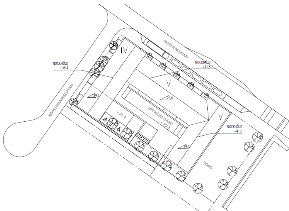
Bild 9 Den tilltänkta bebyggelsens nockhöjd, taklutning och våningsantal. Observera att nockhöjderna är något lägre än detaljplanens högst tillåtna nivåer som är avrundade till närmaste halvmeter för att ge en viss flexibilitet. DinellJohansson
