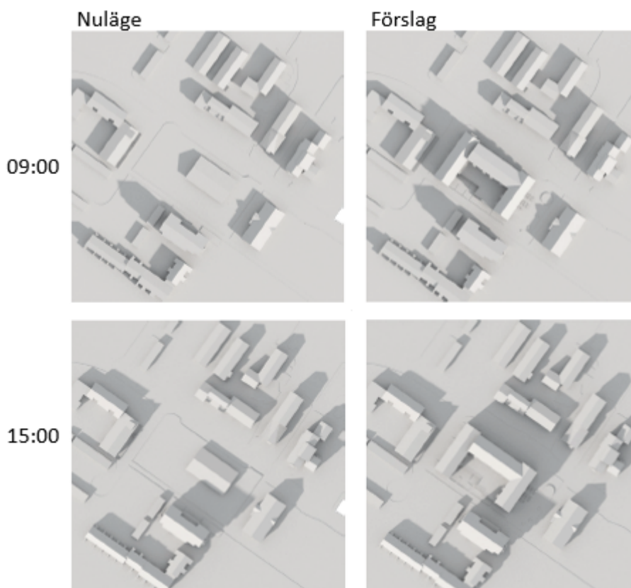
Bild 44 Utdrag ur solstudien som redovisar vårf/höstdagjämning, morgon och eftermiddag vid ett nuläge och enligt förslag. Illustration DinellJohansson
