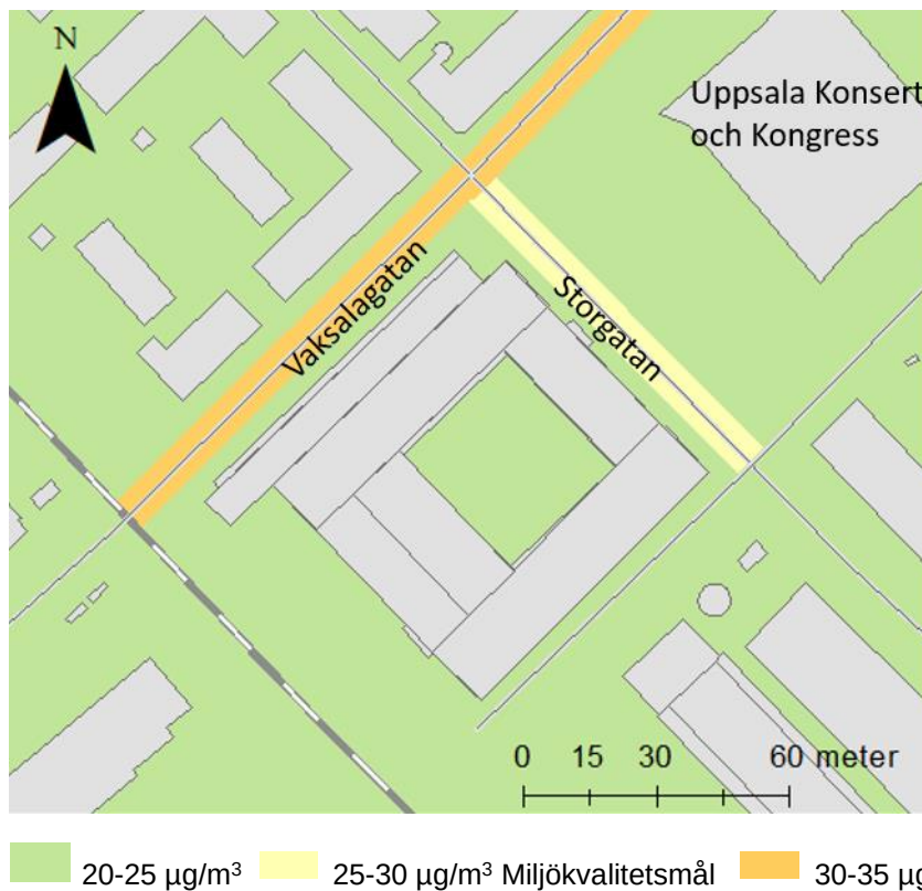
Figur 6. Beräknad dygnsmedelhalt av PM10 ( \mu\text{g}/\text{m}^3 ) under det 36:e värsta dygnet för nollalternativet år 2020. Normvärdet och målvärdet som ska klaras är 50 \mu\text{g}/\text{m}^3 respektive 30 \mu\text{g}/\text{m}^3 .
