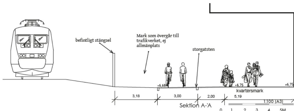
Bild 20 Sektion som visar området mellan järnvägen och den planerade byggnaden. Byggnaden kragar ut över kvartersmarken med en fri höjd på minst 5 meter. Gång- och cykelstråket ska knytas samman med en bro över Vaksalagatan som är en viktig del i det övergripande gång- och cykelnätet. Det kommer även finnas en trappa till Vaksalagatan som fungerar som en genväg till Resecentrum, WSP.
