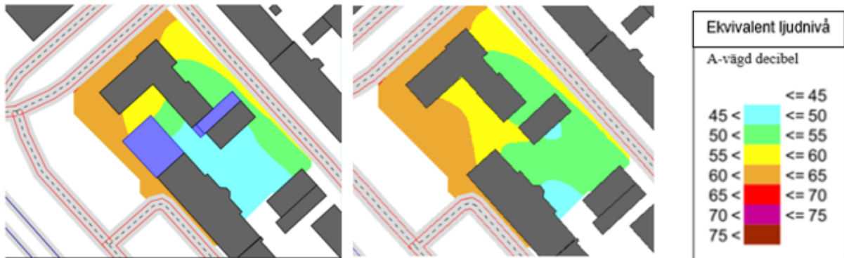
Figur 10. Dagnsekvivalent ljudnivå från väg- och järnvägstrafik, med planerad bebyggelse till vänster, samt utan till höger
