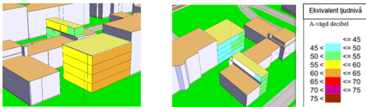
Figur 5. Ekvivalent ljudnivå på fasad från väg- och järnvägstrafik. Bild till vänster är vy från väster och fasader mot spår. Bild till höger är vy från öster.
