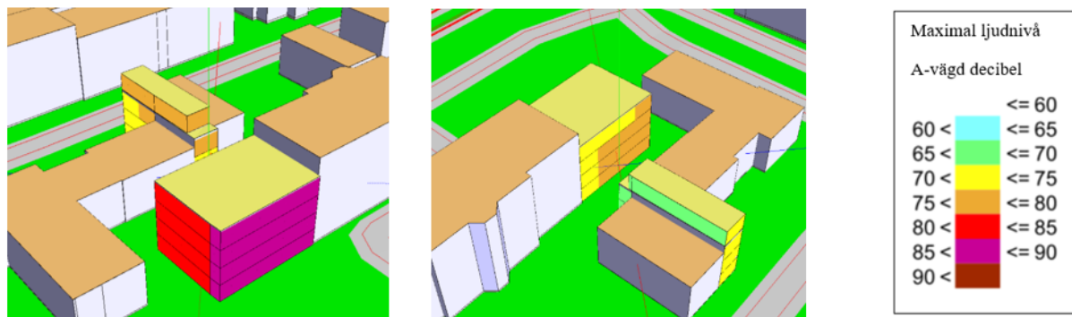
Figur 8. Maximal ljudnivå på fasad från järnvägstrafik. Bild till vänster är vy från väster och fasader mot spår. Bild till höger är vy från öster. För vägtrafik, se bilaga.
