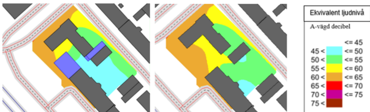
Figur 11. Maximal ljudnivå från järnvägstrafik , med planerad bebyggelse till vänster, samt utan till höger
