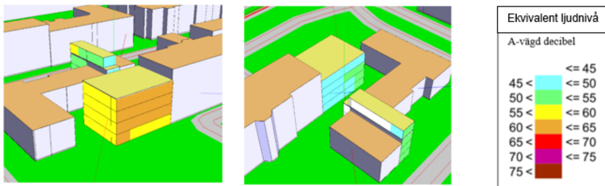
Figur 7. Ekvivalent ljudnivå på fasad från väg- och järnvägstrafik. Bild till vänster är vy från väster och fasader mot spår. Bild till höger är vy från öster.
