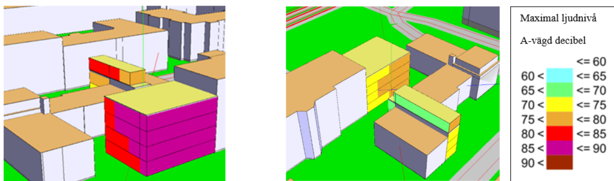
Figur 6. Maximal ljudnivå på fasad från järnvägstrafik. Bild till vänster är vy från väster och fasader mot spår. Bild till höger är vy från öster. För vägtrafik, se bilaga.
