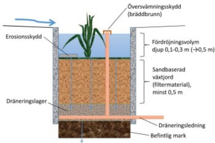
Figur 21: Förslag på uppbyggnad av växtbädd.
