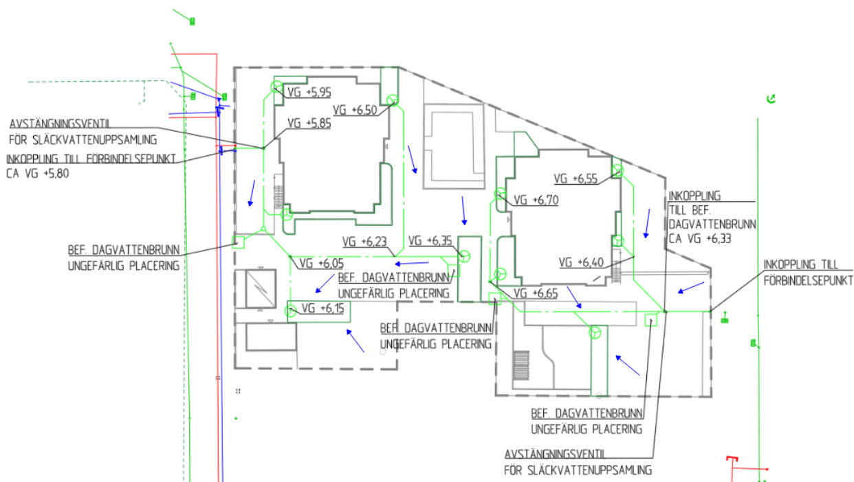
Figur 22: Förslag dagvattenhantering.
