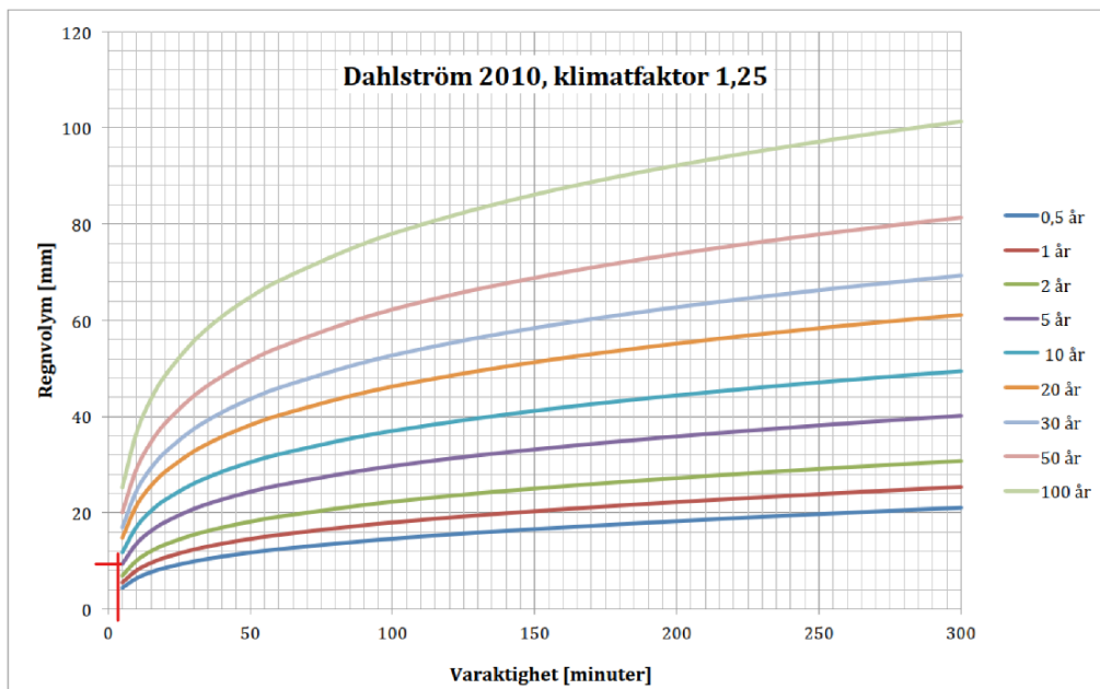
Figur 23: Nederbördsvolym som funktion av varaktighet och återkomsttid (Svenskt vatten P110).
