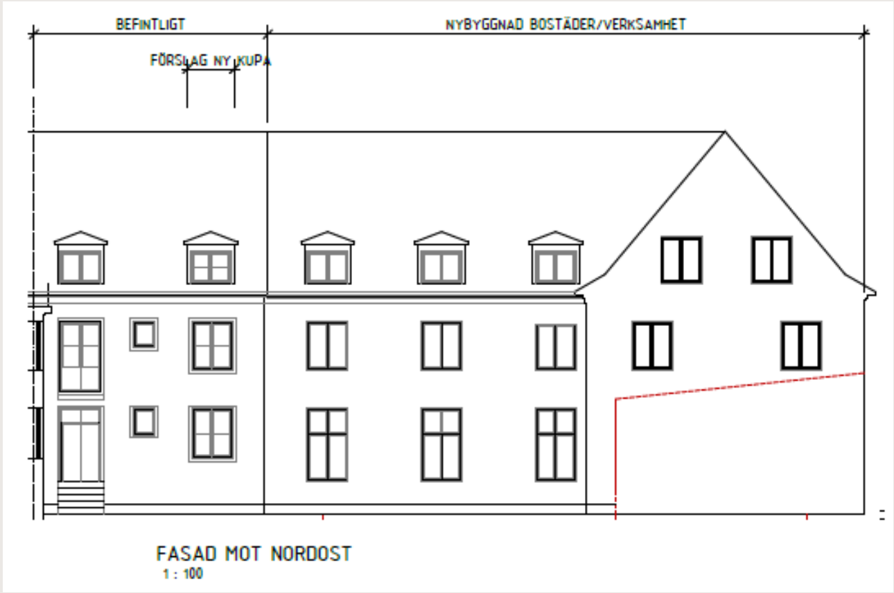
Fasad mot nordost. Ritningen visar mötet mellan Västgötagården och ny byggnad. White arkitekter 2025-05-30.
