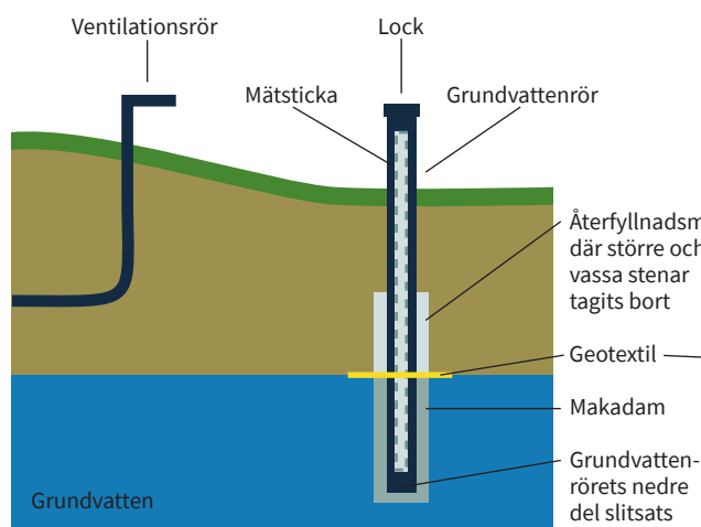
Grundvattenrör vid sidan om bädden.
