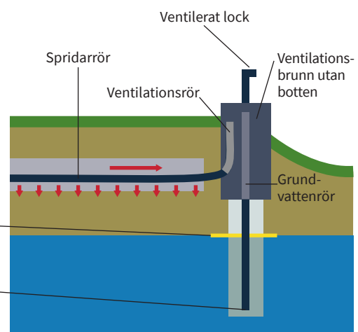
Grundvattenrör i luftningsrör eller ventilationsbrunn.
