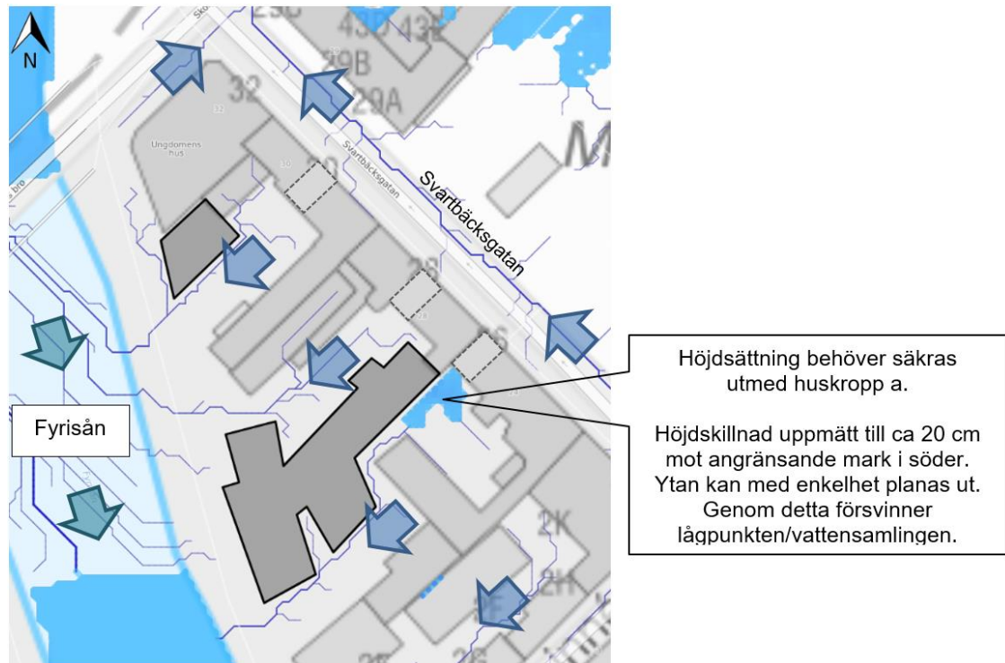
Figur 12. Rinnvägar enligt nuvarande höjdsättning tillsammans med inlagda ytor för planerad byggnation. Portiker mot Svartbäcksgatan är markerat som streckade boxar.
