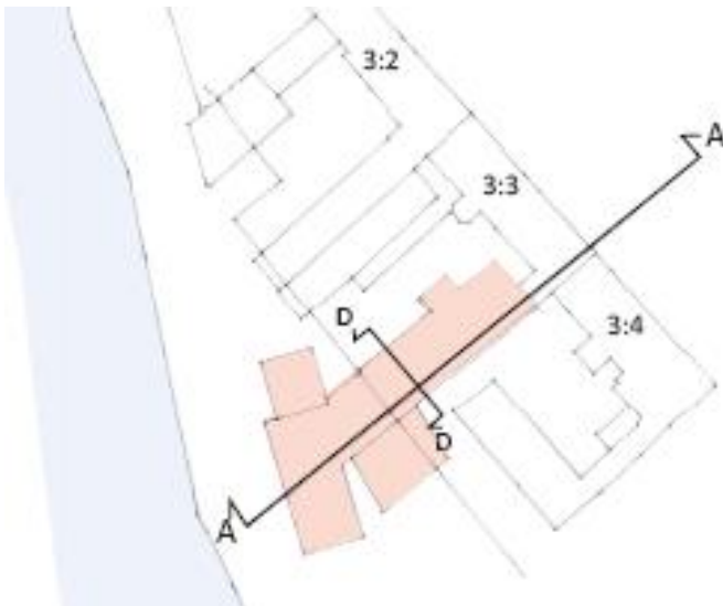
Figur 8. Huvudentré tillgänglighetsanpassad i sektion D-D. Källa: A-sidan
