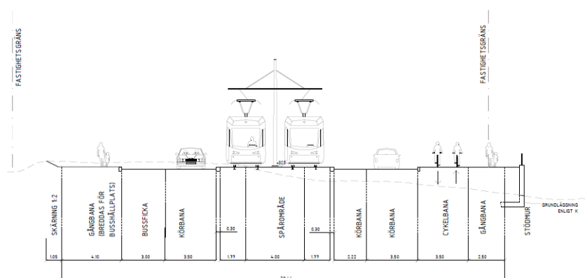
Figur 16 Sektion B17 fastighetsintrång mot sydöst som kräver en stödmur.
