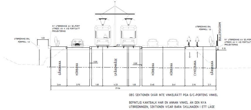
Figur 21 Sektion B24 genom befintlig gc-port.
