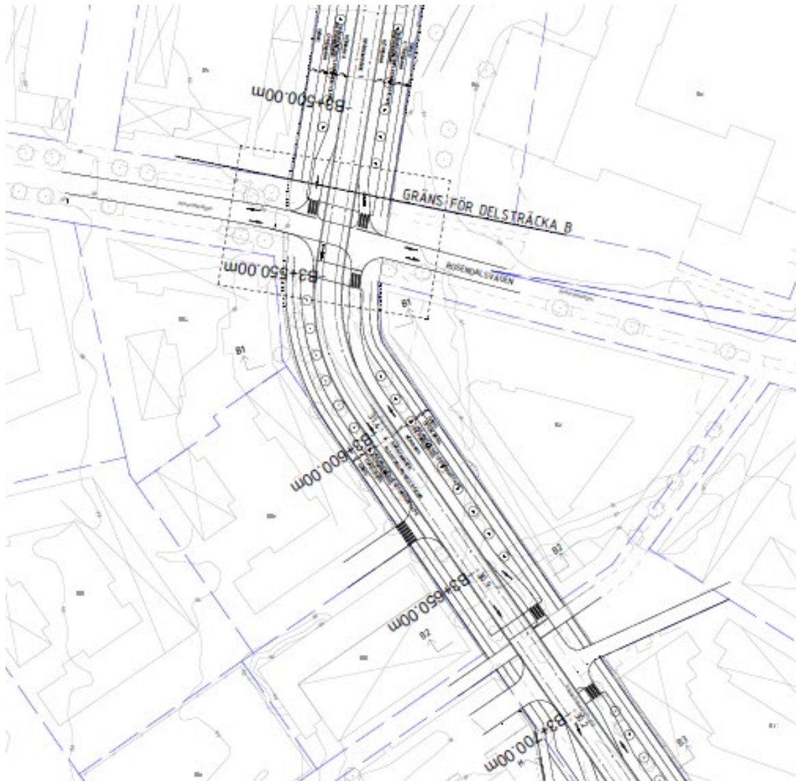
Figur 5 Korsningen Torgny Segerstedts allé/Rosendalsvägen
