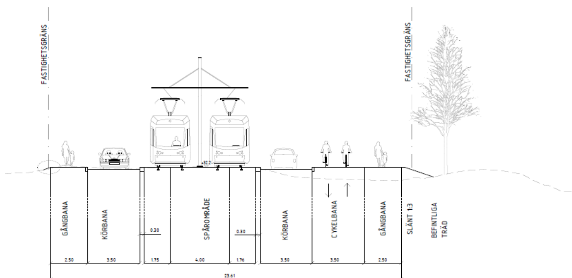
Figur 18 Sektion 19 i höjd med Valsätra IP. Den innersta trädraden med befintliga oxlar kan sparas. En växtbäddsrenovering kommer att behövas för att kunna justera marknivåer inom rotzonen. Raden med stora bokträd utgår dock.
