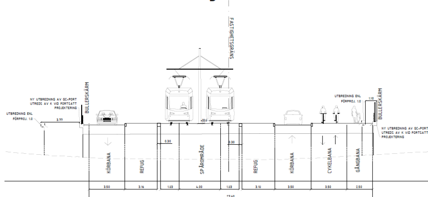
Figur 14 Sektions vid gc-port väster om Slädvägen.
