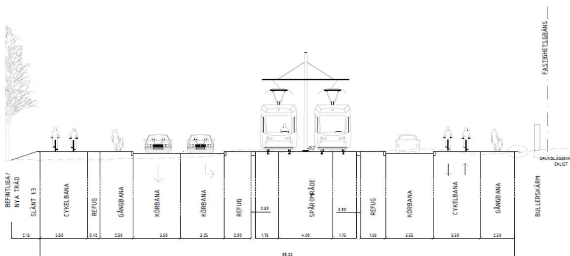
Figur 19 Sektion B22 söder om Bernadottrevägen med intrång i parken på norra sidan
