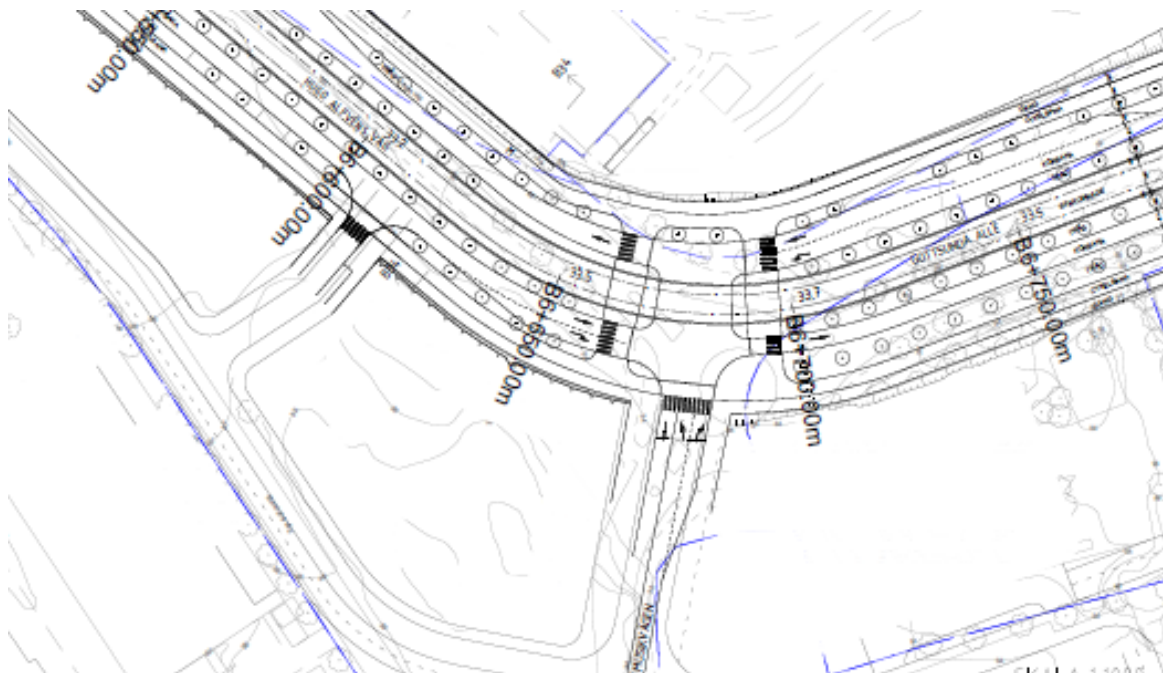
Figur 30 Korsning Hugo Alfvéns väg/Musikvägen/Gottsunda allé med hållplatsläge på Gottsunda allé
