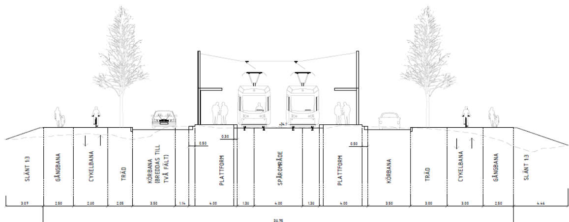
Figur 26 Sektion B29 vid hållplatsläget August Södermans väg.
