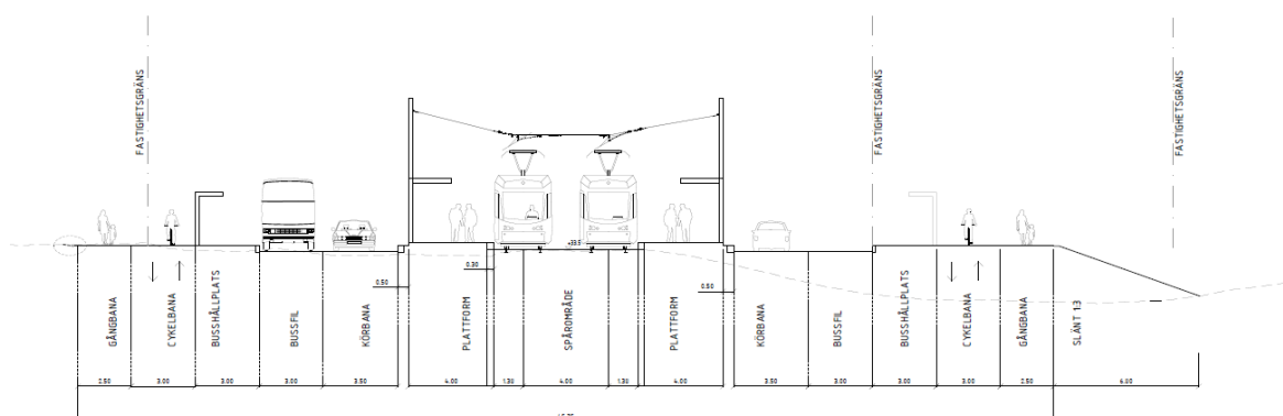
Figur 31 Sektion B34 med hållplatsläge vid Gottsunda C.
