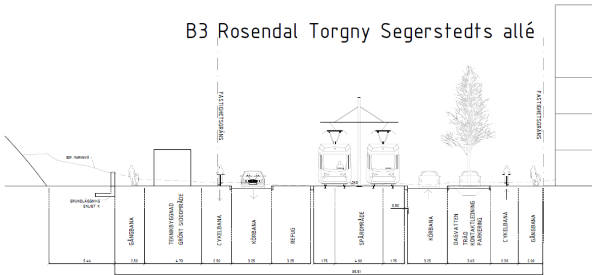
Figur 7 Sektion B3 i höjd med USIF-arena.
