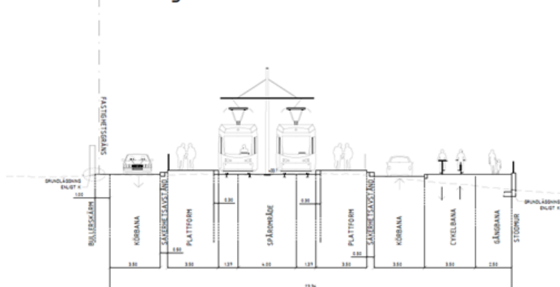
Figur 15 Sektion B14 vid hållplatsläget Valsätraskolan.
