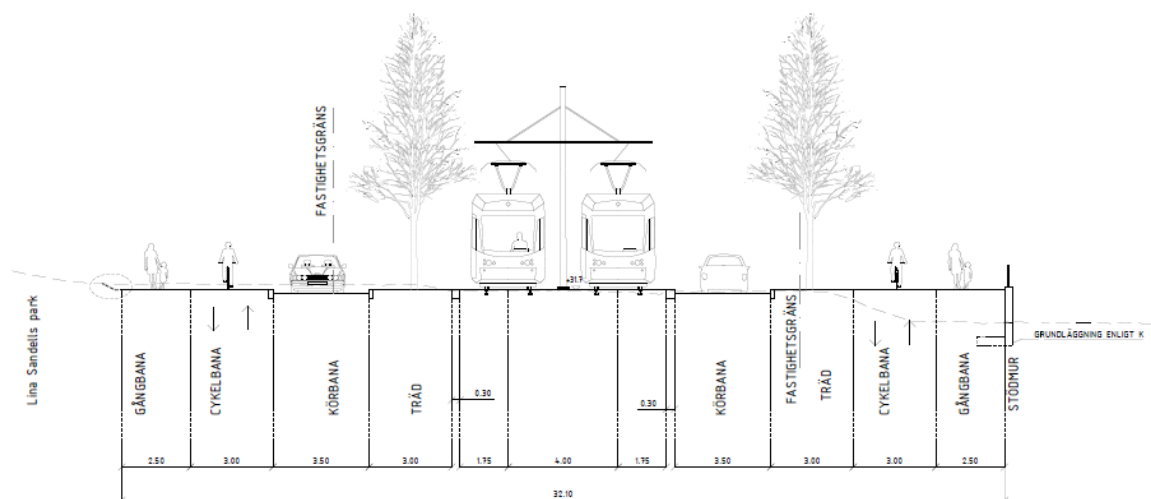
Figur 28 Sektion B30 vid Lina Sandells park.
