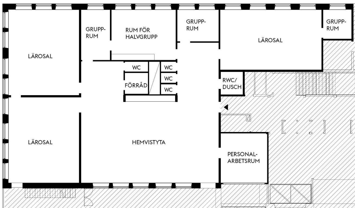
Sluten plan F-3,
