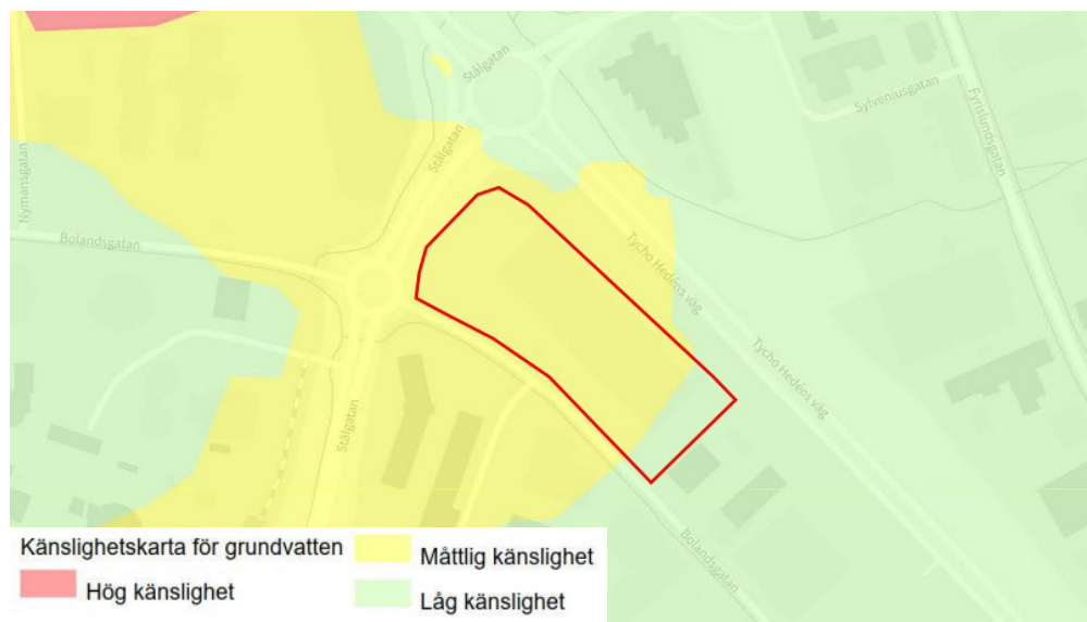
Figur 13, Bilden visar känslighet för grundvatten inom och i anslutning till planområdet. Bilden är från dagvattenutredningen som hör till detaljplanen.
