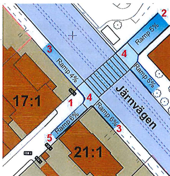
Exempel på plankorsning med rampen placerad intill 21:1 för att kunna behålla angöringen till Dragarbrunn 17:1.
