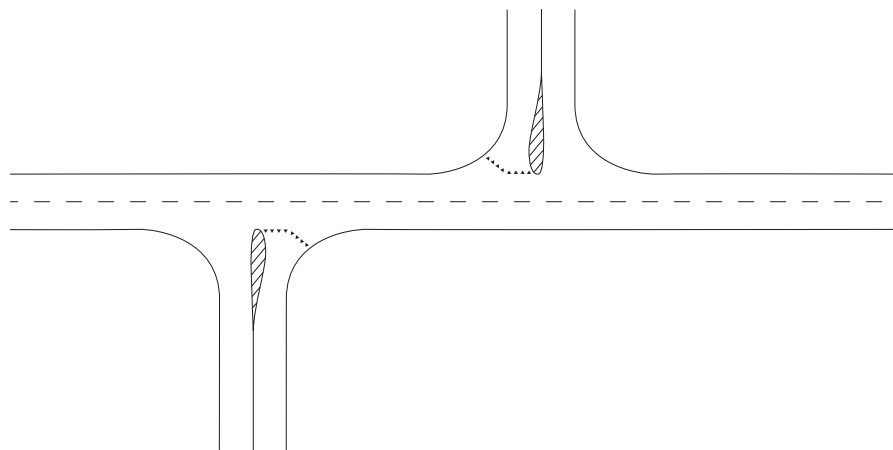
Figur 20 Exempel på förskjuten fyrvägs-korsning utmed väg 635.
