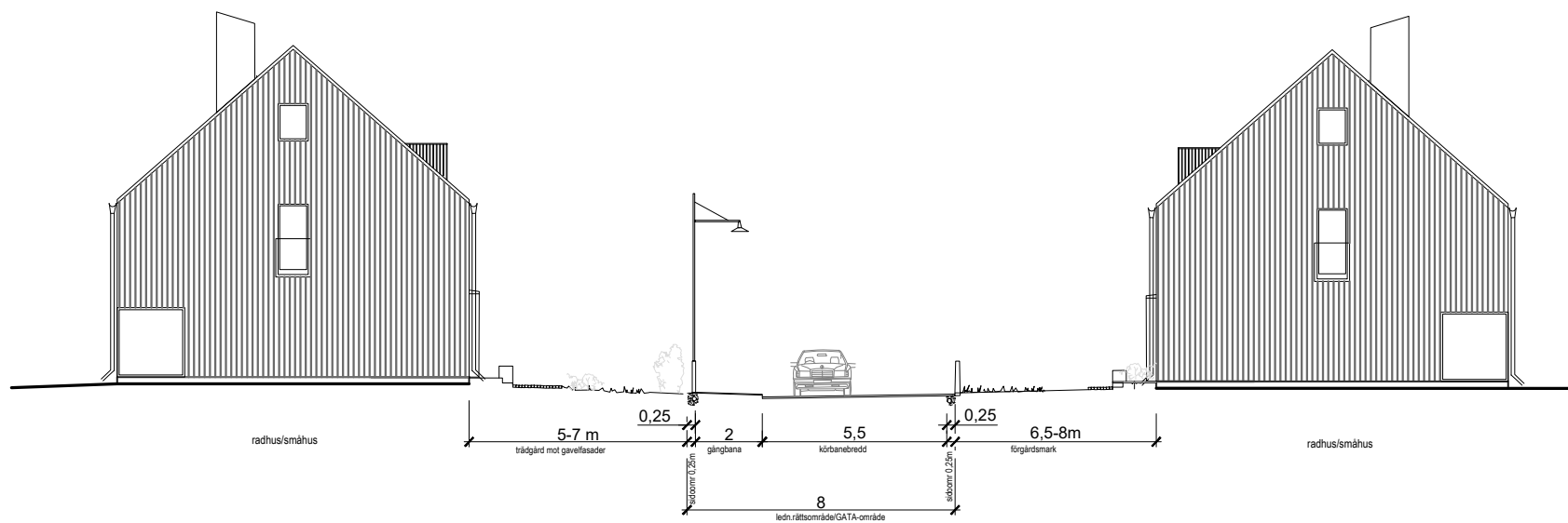
Figur 13 Föreslagen sektion för lokalgator.
