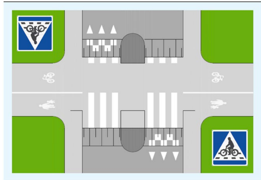
Figur 17 Exempel på hastighetssäkrad gång- och cykelpassage. Utformningen rekommenderas i lokalgatornas korsningspunkter med väg 635. Källa: VGU, Trafikverket.
