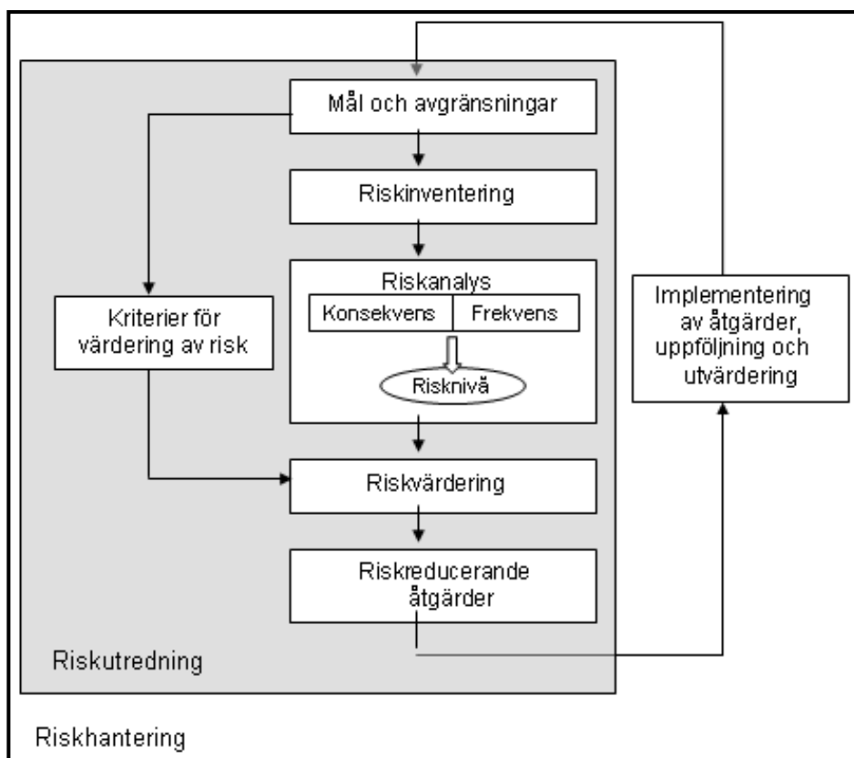
Figur 1. Riskhanteringsprocessen.
