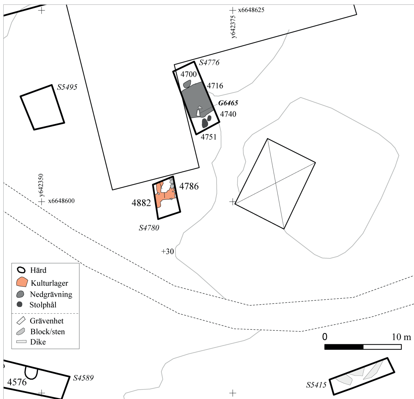
Figur 20. Plan med schakt och arkeologiska objekt i området för ladorna (figur 14). Skala 1:300. Schakt= S+ld, grävenheter= G+ld.
