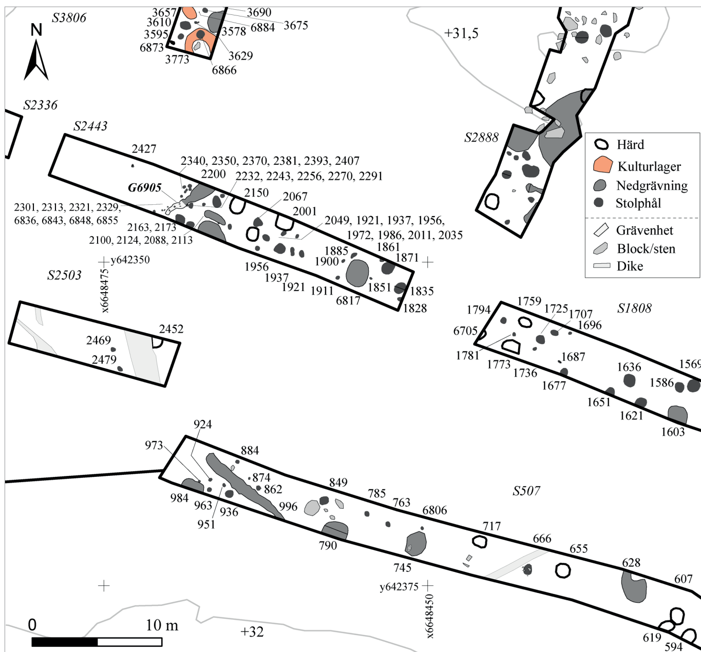
Figur 25. Plan med schakt och arkeologiska objekt sydvästra delen av förundersökningsområdet (figur 14). Skala 1:300. Schakt= S+Id, grävenheter= G+Id. För schakt 2888, se figur 28.
