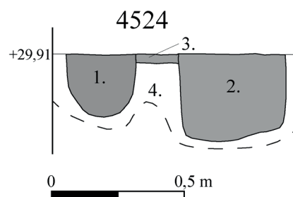
Figur 19. Sektion stolphål 4524. 1: Gråbrun något siltig lera med enstaka kolstänk, br. lera. 2: Som 1 men ljusare, mindre kol. 3: Som 2, möjligen är 6208 igenfylld med samma lager (4524). 4: Ljust brun något siltig lera. (Se även figur 21, schakt 4589). Skala 1:20.
