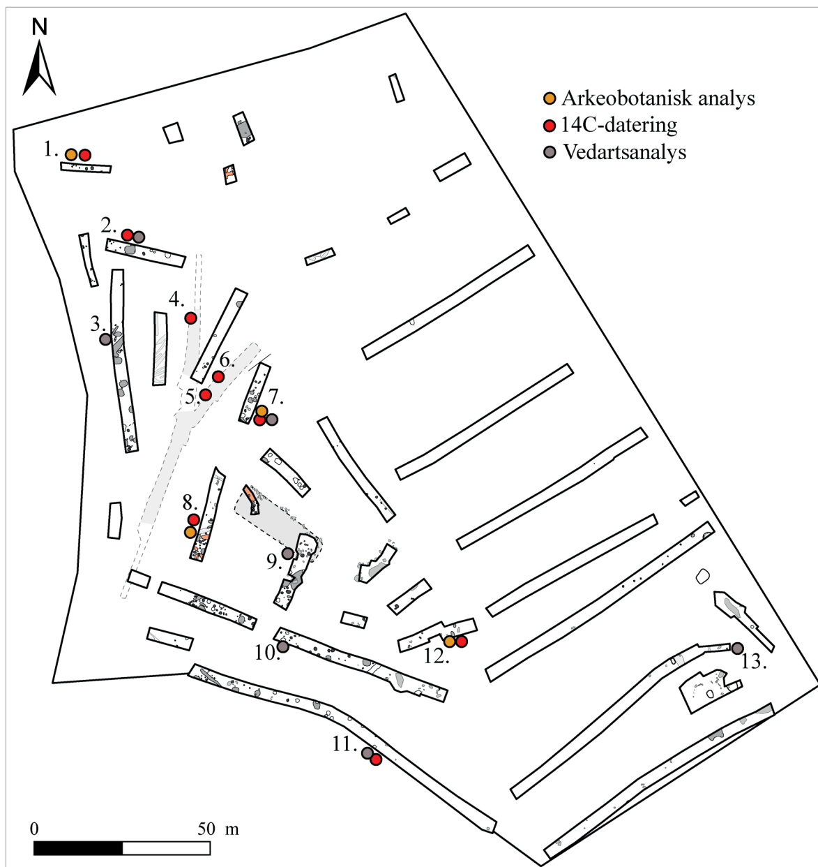
Figur 35. Rumslig fördelning av arkeobotaniska resultat och ^{14}\text{C} -dateringar (inklusive 1992 års dateringar). Littera 1-13 återgår på prov-nr (figur 34, 36) förutom prover från 1992 års undersökning som återgår på Ua-nr (se figur 34, 36). 1: P6590. 2: P6230. 3: P6478. 4: Ua-5957. 5: Ua-5958. 6: Ua-5959. 7: P6524. 8: P6889. 9: P6483. 10: P6676. 11: P6788. 12: P6715. 13: P6198. Skala 1: 1 500.
