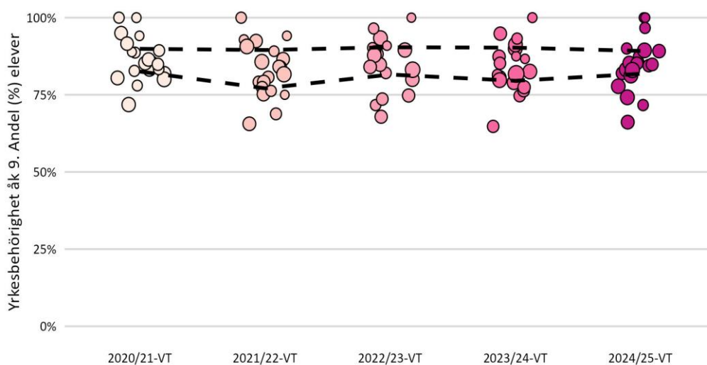
Diagram 23: Andel elever behöriga till yrkesprogram per skola: Årskurs 9, kommunal skola 2021–2025. Varje bubbla motsvarar en skola, storleken på bubblan beror på antal elever, de streckade linjerna är första och tredje kvartilen.
