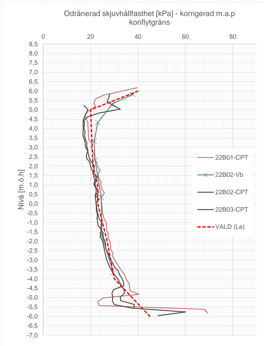
Figur 4. Sammanställning av odränerade skjuvhållfastheten samt valda värden plottad mot nivå.
