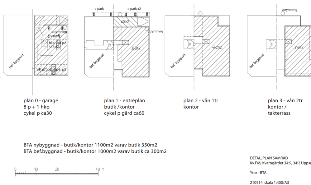
Bild 40 Planritningar över samtliga våningsplan (VESPR AB 2021-09-30).
