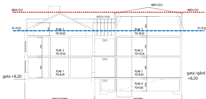
Bild 9 Sektion och höjder. Sektionen går genom Pantbankshuset och den nya tillbyggnaden sett från fasaden som vänder sig mot Salagatan. Den blåa linjen visar byggnadernas takfot. Den röda linjen visar pantbankshusets nockhöjd (ritning: VESPR AB).
