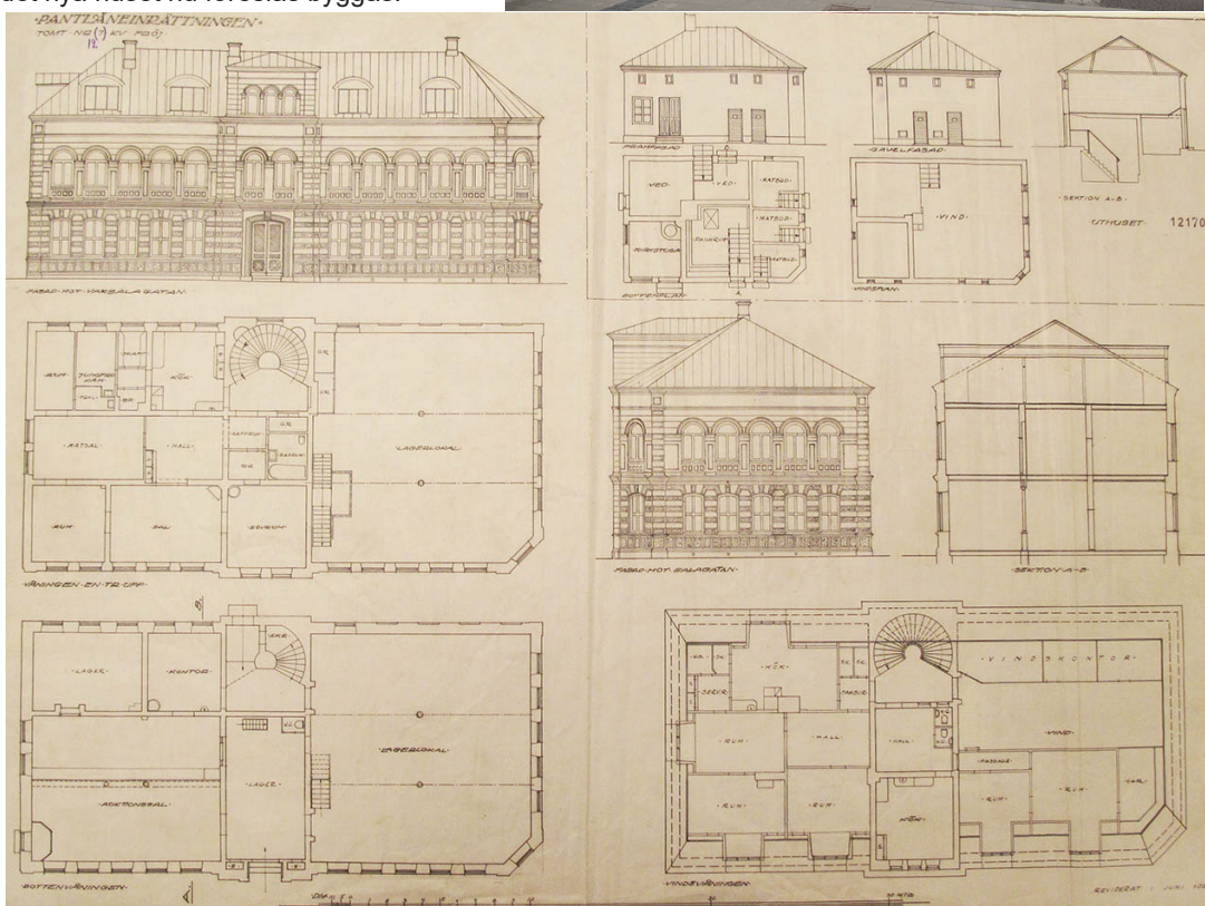
“Pantlåneinrättningen”. Bygglövsritning från 1932 gällande inredande av vind och ändring av gårdshus. Uppsala stadsarkiv.
