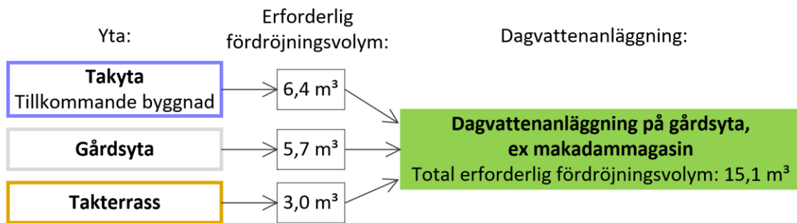
Figur 14. Flödesschema för föreslagen dagvattenhantering inom utredningsområdet. Ytor och dagvattenanläggningar är färgsatta på samma sätt som avvattningsplanen i Figur 15.
