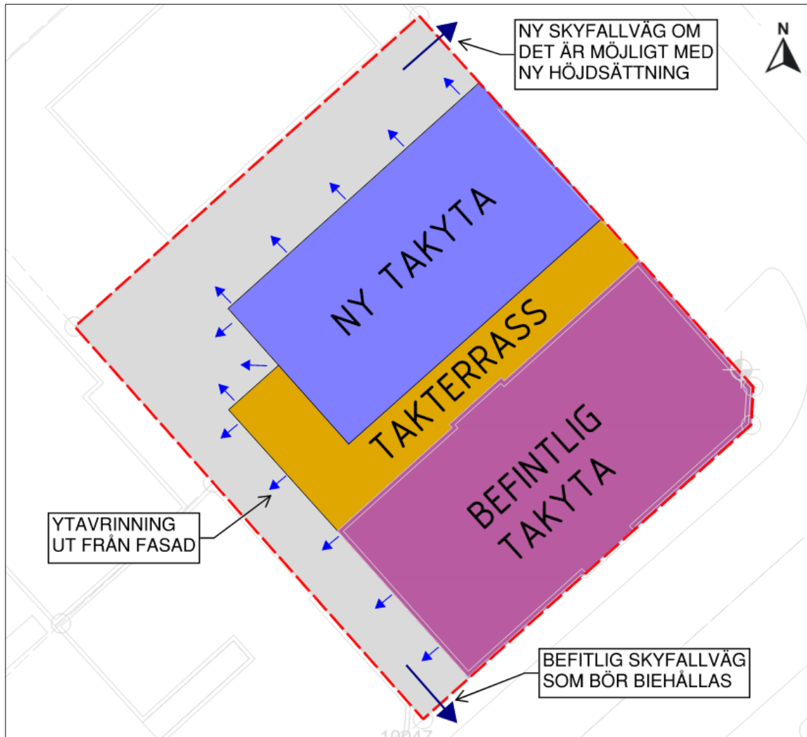
Figur 17. Skyfallsplan ny planerad situation. Om möjligt bör höjdsättningen av gårdsytan i och med den planerade exploateringen utformas för att leda skyfallsvatten enligt flödespilar.
