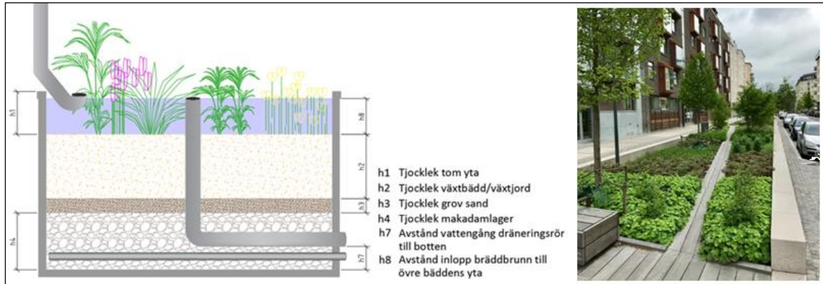
Figur 13. Principskiss av växtbädd och foto av en nedsänkt växtbädd (Structor Uppsala AB, 2017).
