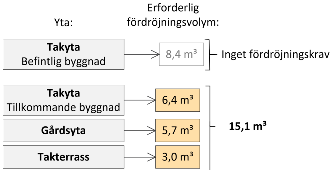
Figur 11. Flödesschema för erforderliga fördröjningsvolymen inom utredningsområdet.
