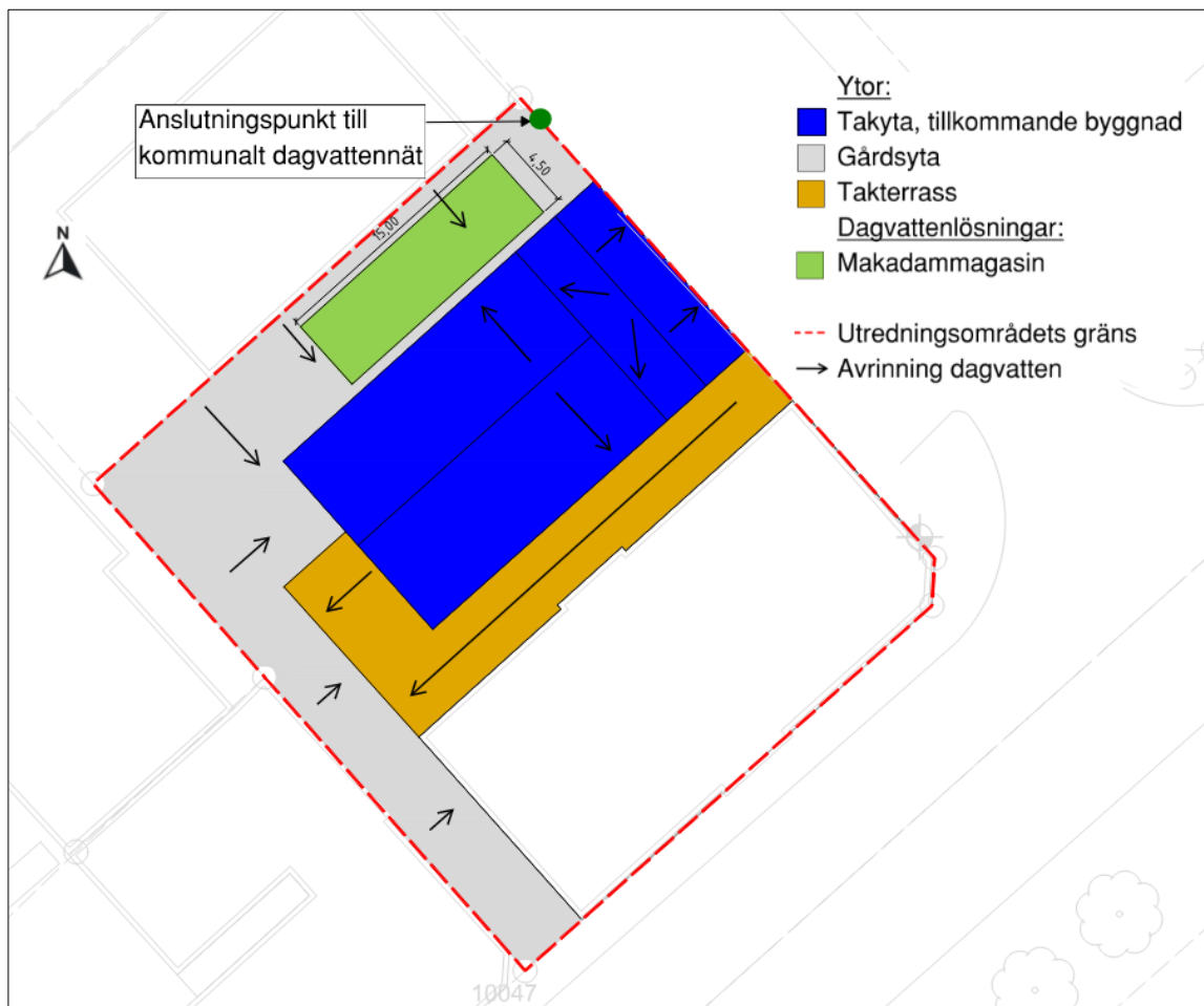
Figur 15. Föreslagen systemlösning för dagvattenhantering inom utredningsområdet. Ytor och dagvattenanläggningar är färgsatta på samma sätt som flödesschemat i Figur 14.
