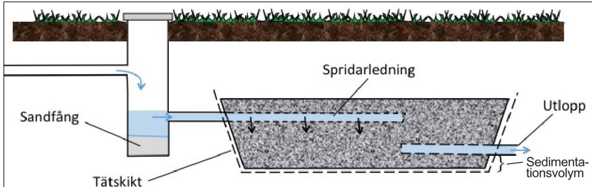
Figur 12. Typillustration av makadammagasin (Stockholm Vatten och Avfall, 2019).
