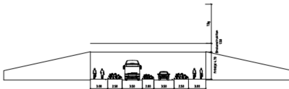
Sektion 0/410 Tunnel Alternativ
