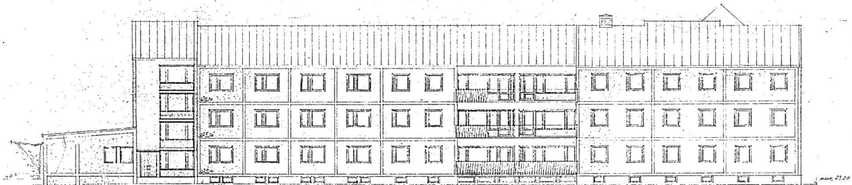
Hus A, fasadritning bygglovsansökan, originalritning K W Ottossons arkitektkontor Nacka
