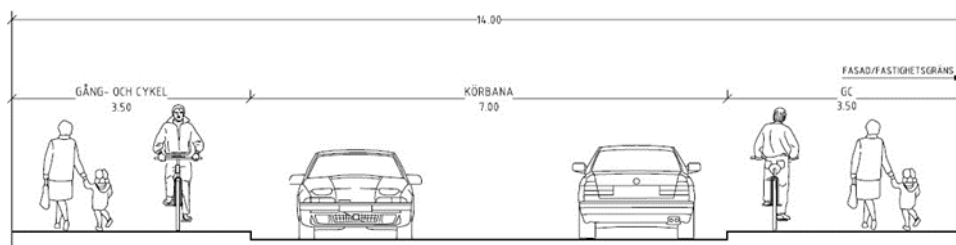
Bild 40 Gatusektion som redovisar möjlig sektion för Granitvägen. (WSP)
