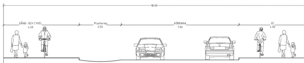
Bild 39 Gatusektion som redovisar möjlig sektion för Eriksbergsvägen. (WSP)
