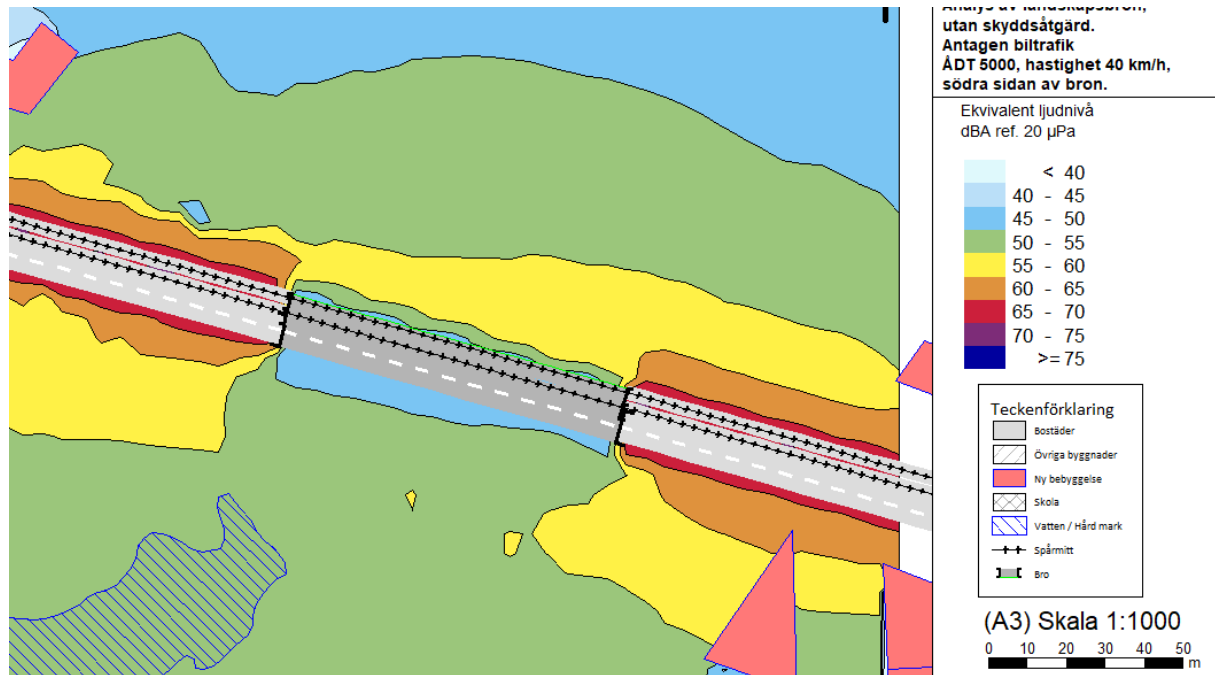
Figur 16 Ekvivalent bullernivå 1,5 m ovan mark från väg- och spårtrafik vid landskapsbron/faunapassagen. Ingen skyddsåtgärd. 55 dBA överskrids norr om bron. Det skräpperade området nere till vänster är Stordammen.
