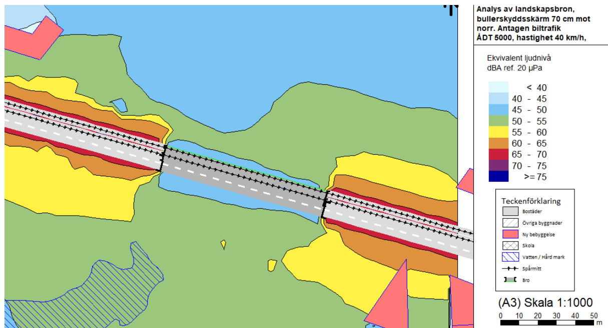
Figur 17 Ekvivalent bullernivå 1,5 m ovan mark från väg- och spårtrafik vid landskapsbron/faunapassagen. Med 70 cm bullerskärm längs brons norra kant. Det skräpperade området nere till vänster är Stordammen.
