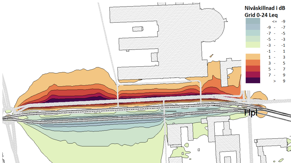
Figur 9 Skillnad mellan den alternativa sträckningen och huvudalternativet. Figuren visar ekvivalentnivå för den alternativa sträckningen minus ekvivalentnivå för huvudalternativet
