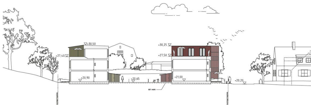
Sektion genom planområdet som visar hur gestaltningsförslaget förhåller sig till närmiljön. Illustration: DinellJohansson.
