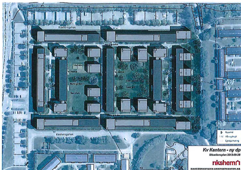
Situationsplan med föreslagna nya byggnader i ljusgrått och befintliga byggnader i mörkgrått. Illustration utförd av Hans Berndtsson Arkitektkontor AB. Observera att norr inte är orienterat uppåt i illustrationen.
