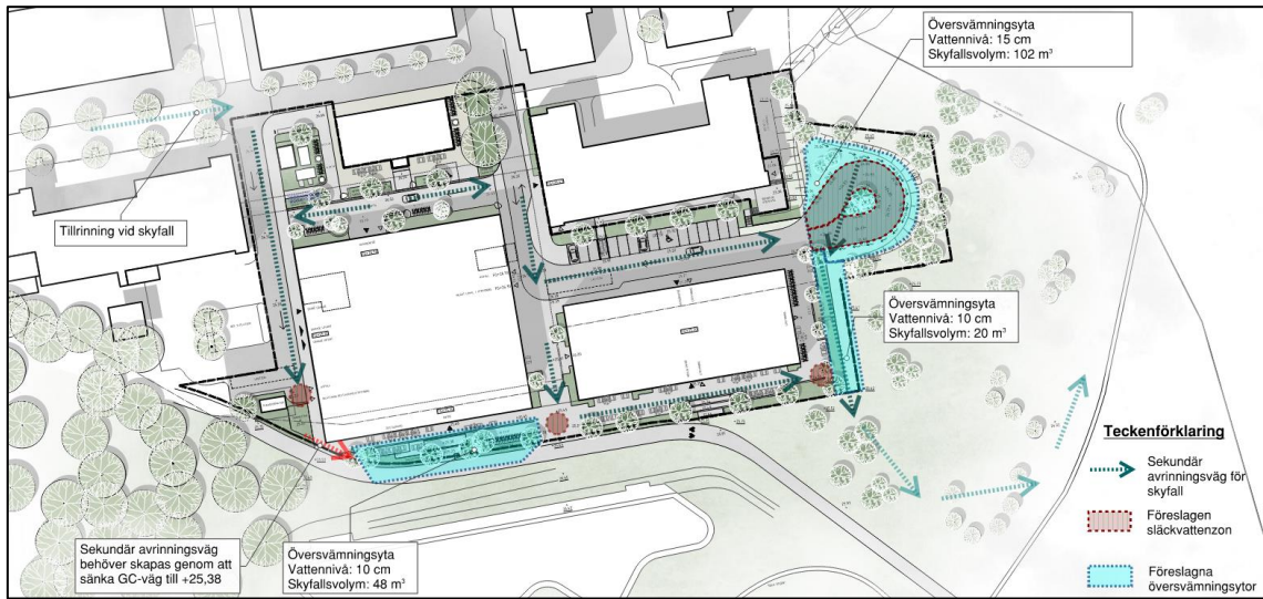
Figur 8-4. Föreslagna sekundära avrinningsvägar inom och intill utredningsområdet, tillsammans med föreslagna översvämningsytor. Nedströms förskola är lokaliserad nordöst om utredningsområdet.
