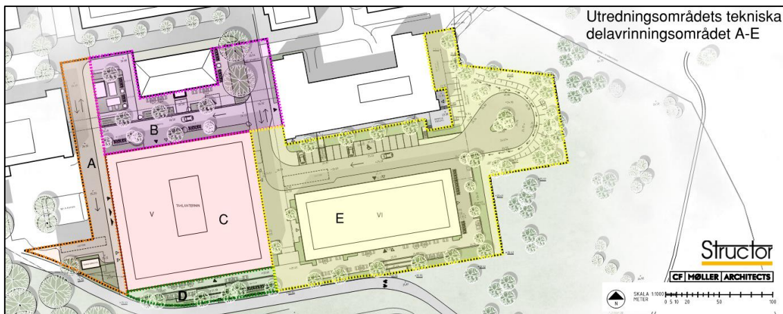
Figur 4-6. Planerade tekniska delavrinningsområden A – E inom utredningsområdet.
