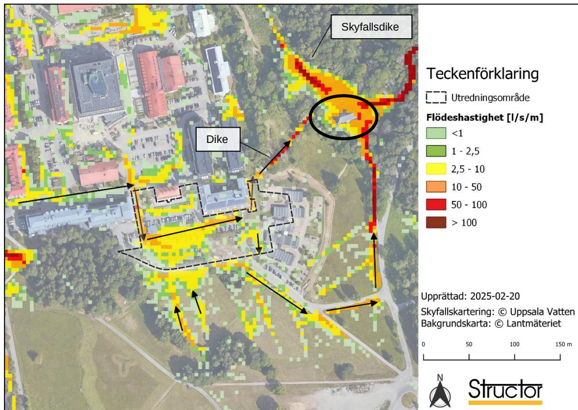
Figur 8-2. Flödesvägar vid dimensionerande 100-årsregn inom och omkring utredningsområdet, enligt Uppsala Vattens skyfallskartering. Befintlig förskola nedströms utredningsområdet är markerad med en svart ellips. Observera att den temporära förskolan vid utredningsområdets östra gräns har monterats ned.
