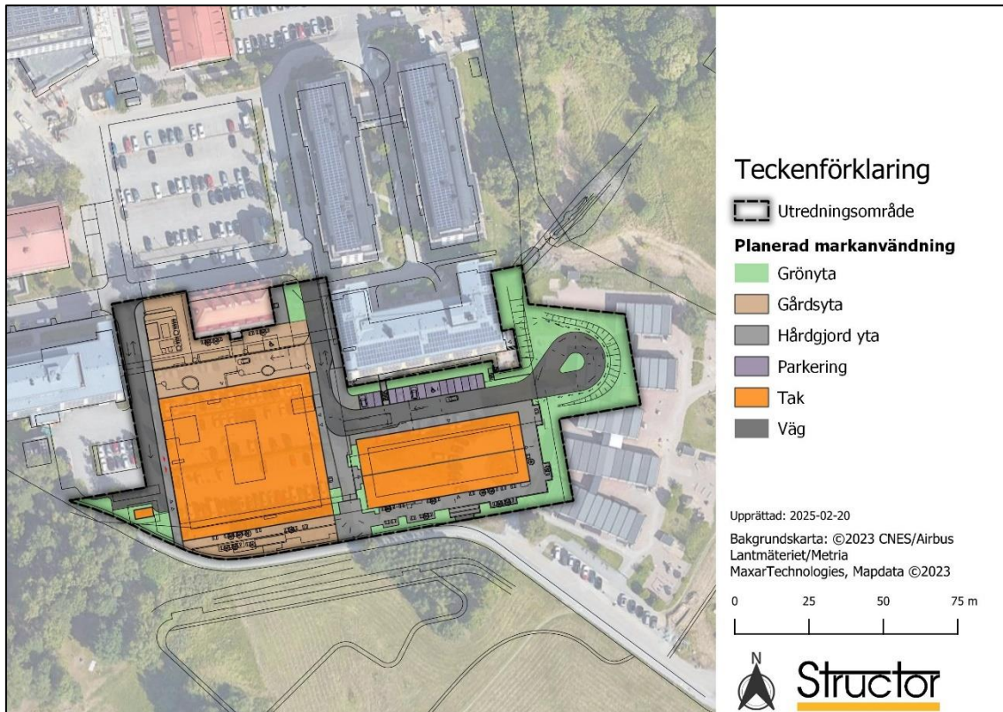
Figur 4-2. Planerad markanvändning inom utredningsområdet (situationsplan daterad 2025-01-28).
