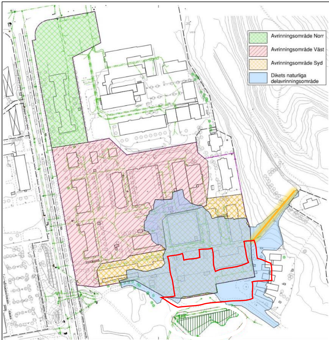
Figur 4-5. Tekniska och naturliga avrinningsområden i Uppsala Science Park och ungefärligt utredningsområdet (röd linje). Nordöst om utredningsområdet finns ett dagvattendike (tjock orange linje), dit avrinning sker från avrinningsområdet till nedströms skyfallsdike, som leder dagvattnet vidare till Fyrisån. I figuren visas den tidigare förskolebyggnaden, numera nedmonterad. Figuren är modifierad från PM Dagvatten Kronåsen Uppsala, upprättad av Structor Mark Uppsala (2023).
