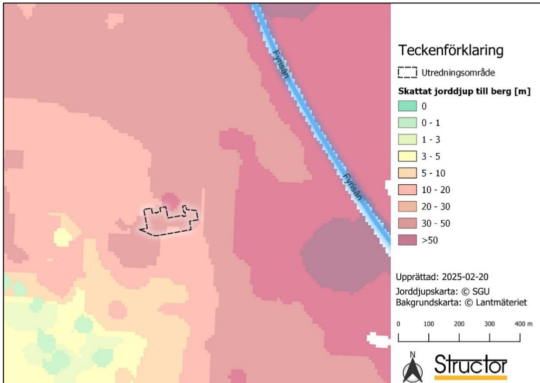
Figur 4-4. Jorddjup enligt SGU:s jorddjupskarta med en upplösning på 10x10 m (SGU 2023), hämtad från SGU:s WMS tjänst. Utredningsområdet har markerats med en svartstreckad linje.
