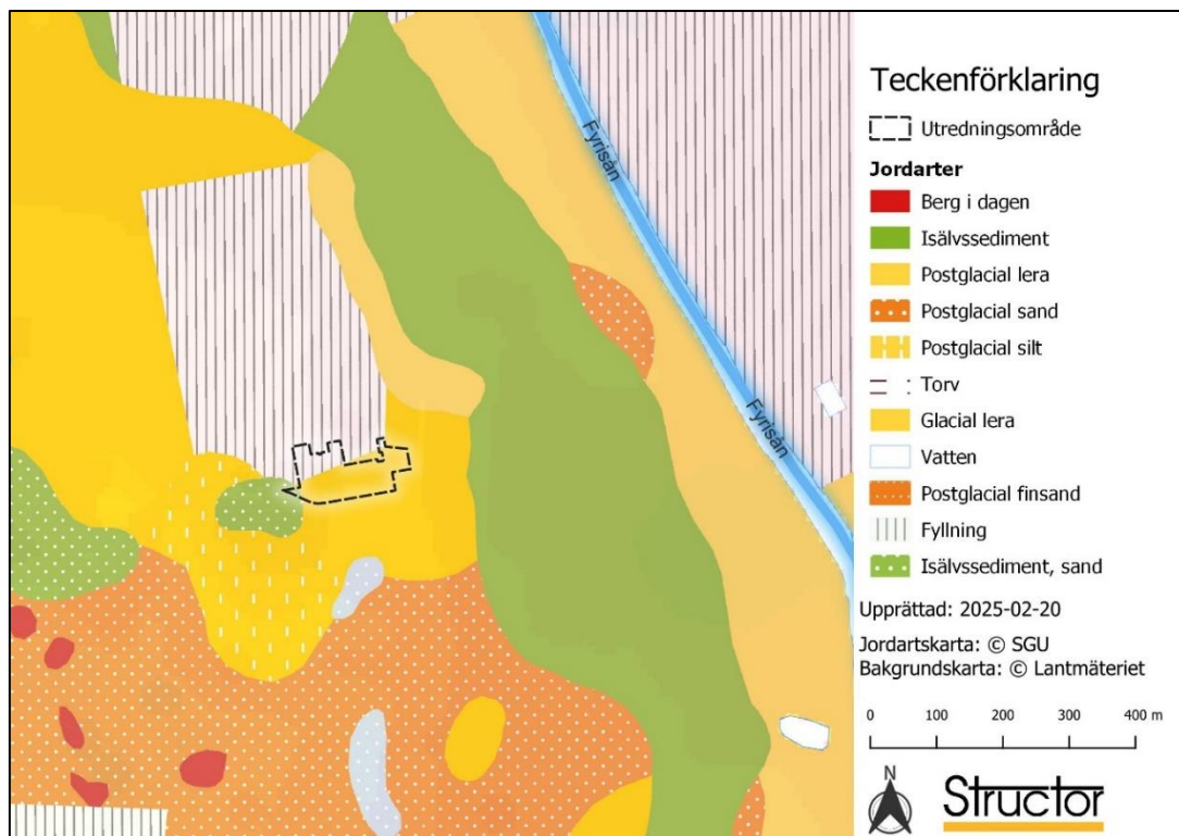
Figur 4-3. Jordarter enligt SGU:s jordartskarta i skala 1:25 000 - 100 000 (SGU 2023), hämtad från SGU:s WMS-tjänst. Utredningsområdet har markerats med en röstreckad linje.
