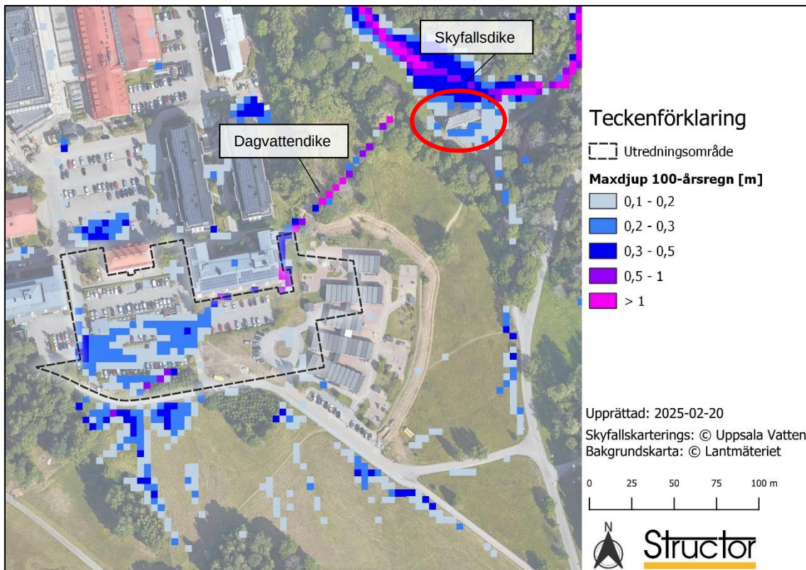
Figur 8-1. Maxdjup vid dimensionerande 100-årsregn inom och omkring utredningsområdet, enligt Uppsala Vattens skyfallskartering. Befintlig förskola nedströms utredningsområdet är markerad med en röd ellips. Observera att den temporära förskolan vid utredningsområdets östra gräns har monterats ned.
