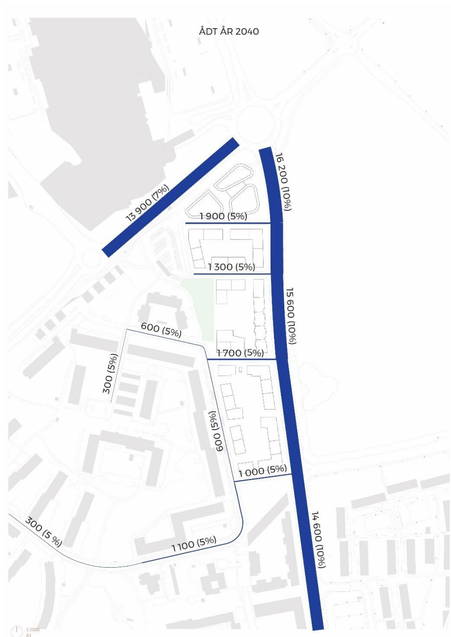
Figur 9. Framtidens trafikflöden (ÅDT). Siffran i parantes avser andel tung trafik.
