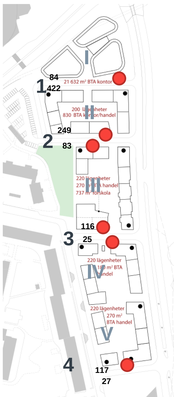
Figur 11. Parkeringar (röda cirklar) i varje område I-V samt anslutningsvägar markerade 1–4. Svarta tal anger flöde per riktning under eftermiddagens maxtimme.
