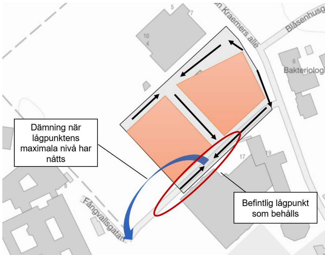
Figur 15. Förslag på framtida skyfallshantering. Svarta pilar visar yttliga skyfallsvägar. Höjdsättning bör efterlikna befintliga höjder, befintlig lågpunkt på Fångvallsgatan behöver behållas och tillåts bräddas till sydväst såsom idag.
