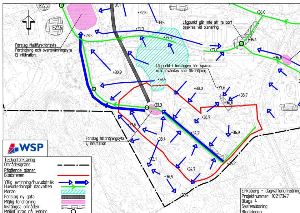
Figur 16. Systemlösning för delområdet som innefattar Blodstenen. Se även bilaga 4.
