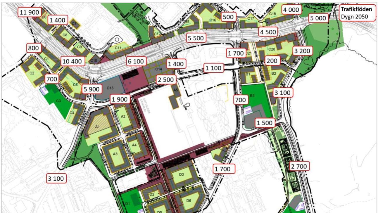
Figur 5. Trafikflöden (ÅDVT) 2050
