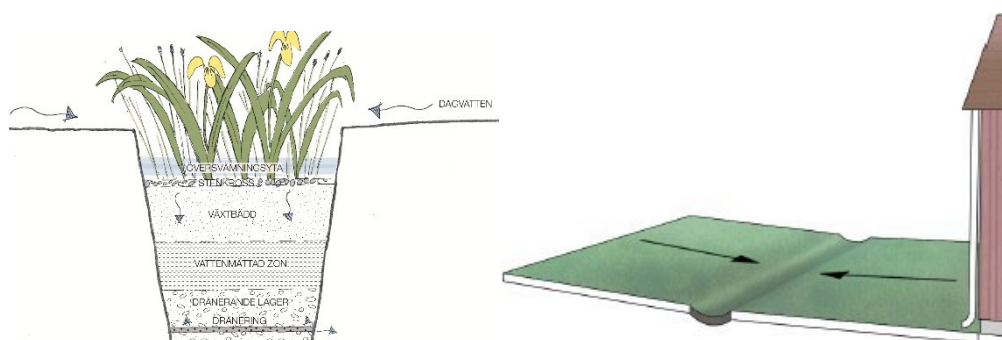
Figur 16, till vänster principskiss över en nedsänkt växtbädd (illustration: Norconsult). Till höger principskiss över ett Svackdike (Illustration: Norconsult).
